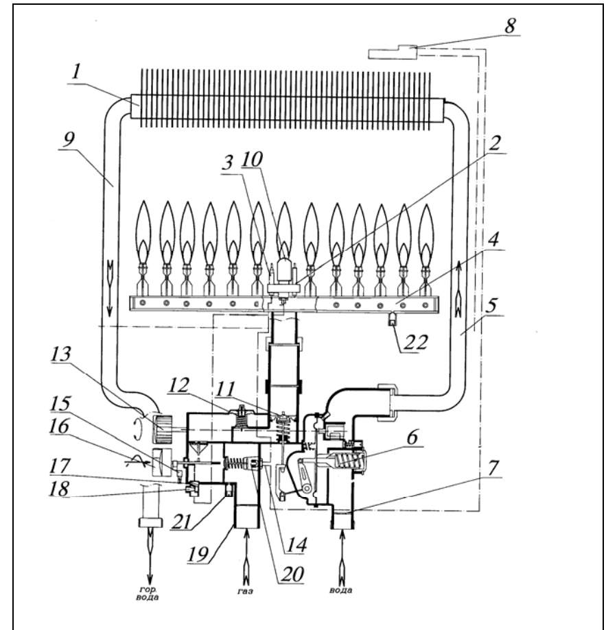
1-теплообменник; 2-запальная свеча; 3-термопара; 4-основная горелка; 5-входная водяная труба; 6-регулятор водяной; 7-фильтр водяной; 8-датчик контроля тяги; 9-выходная водяная труба; 10-запальная горелка; 11-газовый клапан; 12-регулятор давления газа; 13-ручка регулятора температуры воды; 14-термоэлектрический провод; 15-пьезоэлемент; 16-ручка розжига и регулировки мощности; 17-газовый фильтр запальной горелки; 18-винт регулировки пламени запальной горелки; 19-газовый фильтр; 20-электромагнитный клапан; 21-штуцер контроля давления газа перед аппаратом; 22-штуцер контроля давления газа перед соплами горелки
