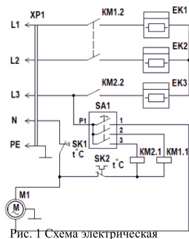
Рис. 1 Схема электрическая
