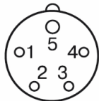
Рис. 2 Схема контактов на вилке
