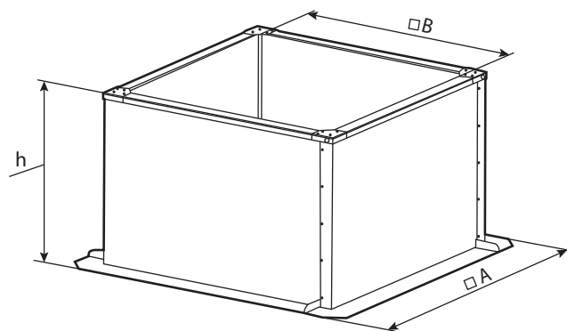
Рисунок 2. Монтажный стакан
