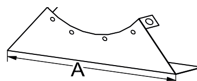
Рисунок 11. Опора вентилятора
