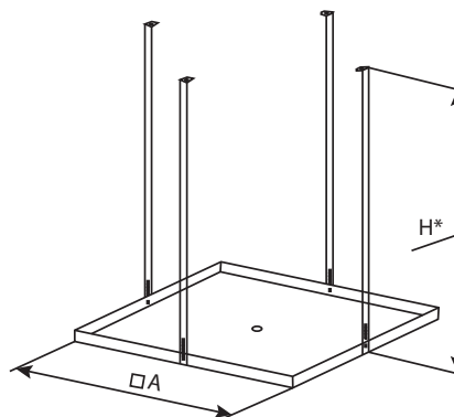
Рисунок 4. Поддон
