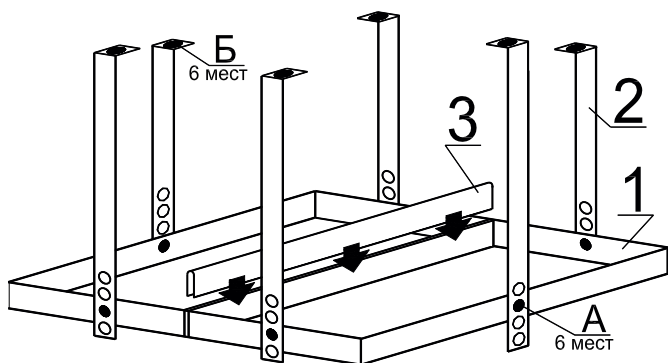
Рисунок 17. Монтаж поддона
