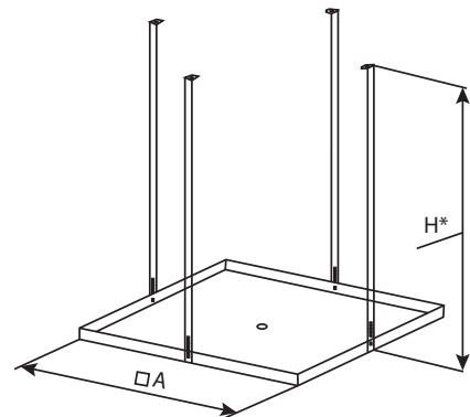
Рисунок 5. Поддон
