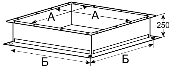
Рисунок 4. Адаптер для противопожарных клапанов
