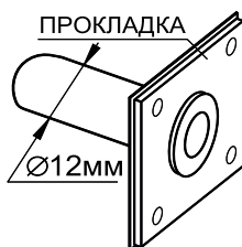
Штуцер с уплотнительной прокладкой (1 шт.)
