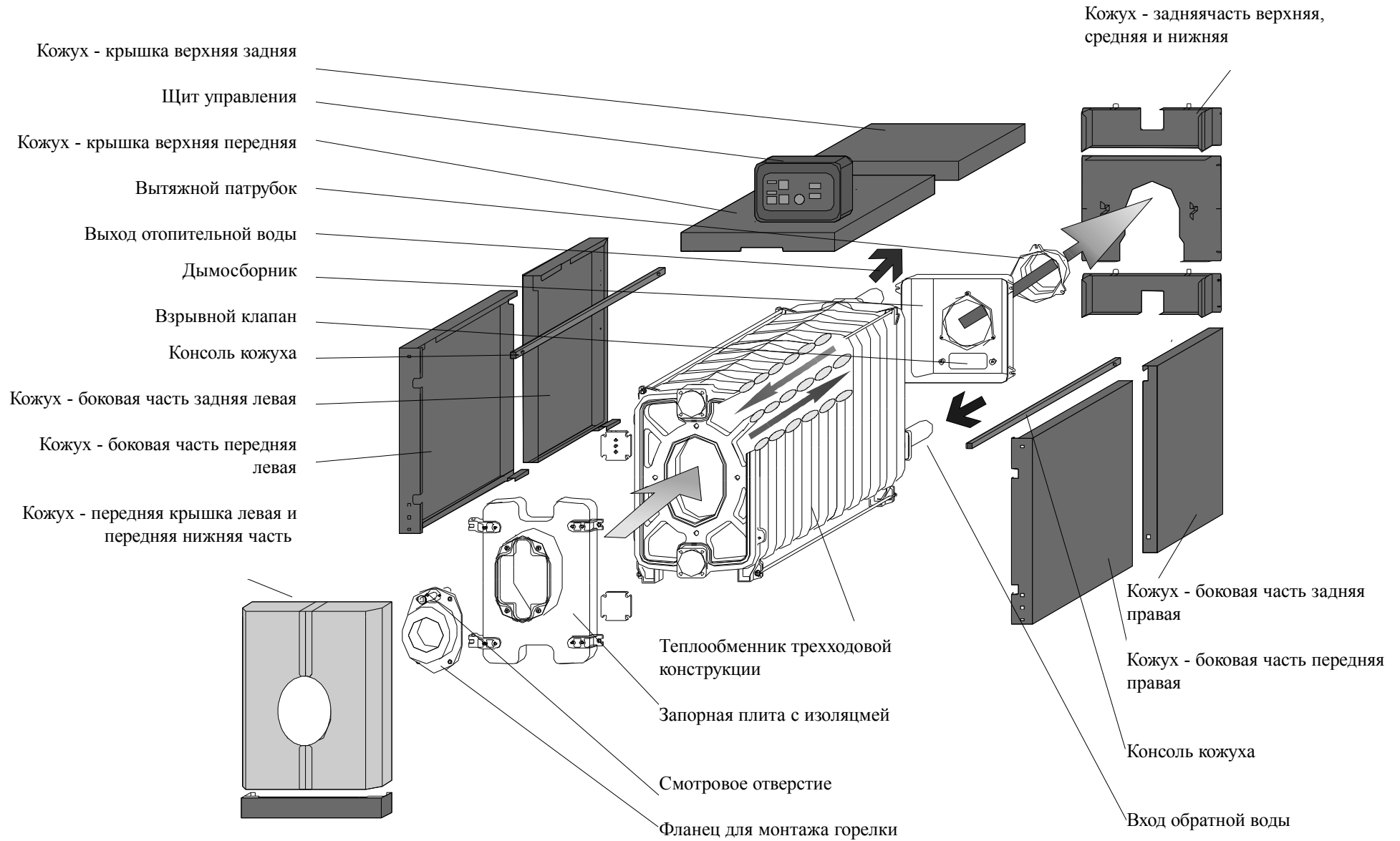
Рис. 1 Схема котла
