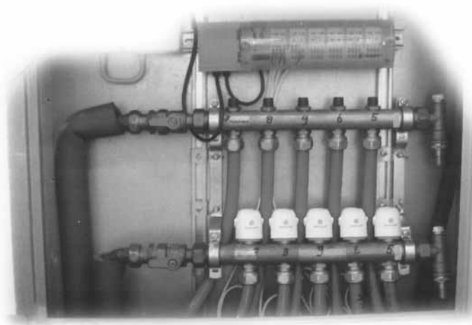
Место монтажа в распределительном шкафу отопительного контура
