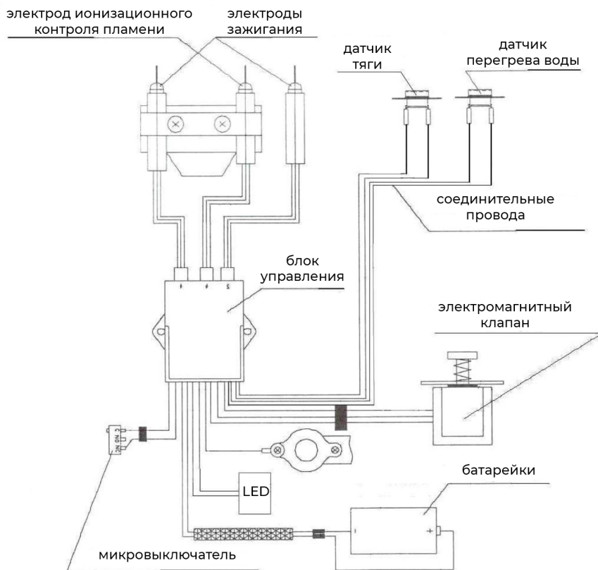
Рис.2. Схема электрическая
