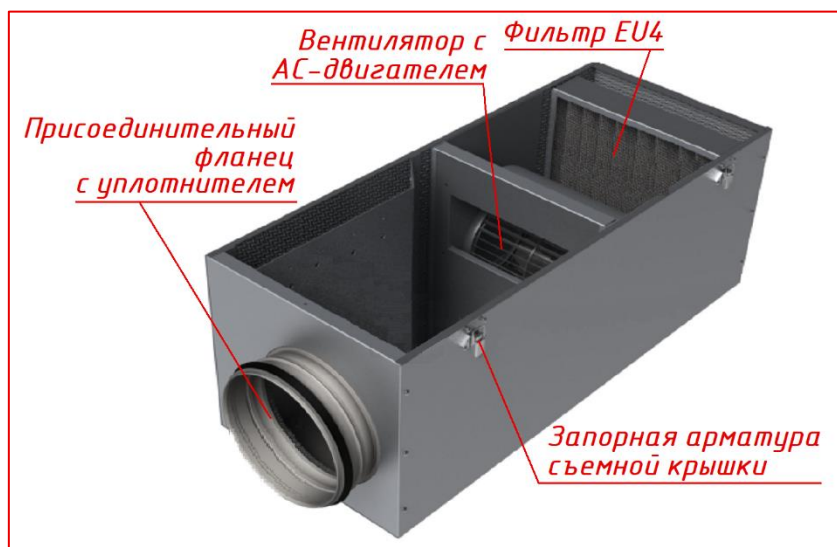
MIRAVENT VA 400 AC
