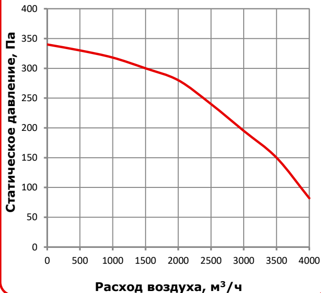
MIRAVENT VA 4000 EC
