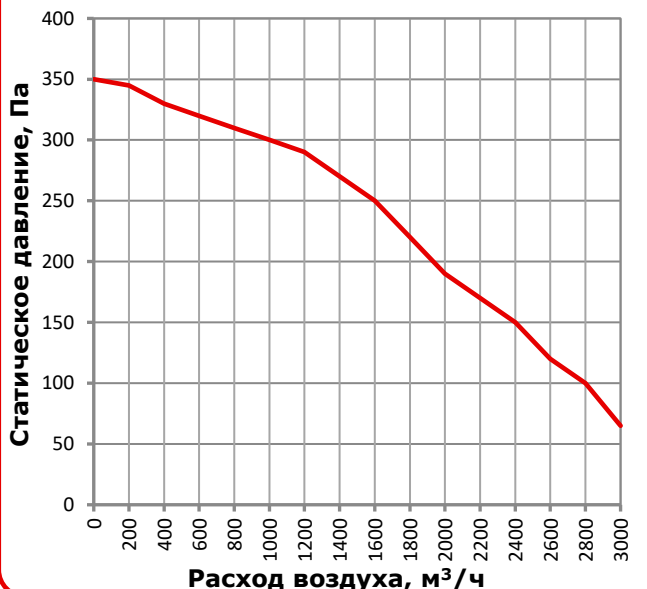
MIRAVENT VA 3000 EC
