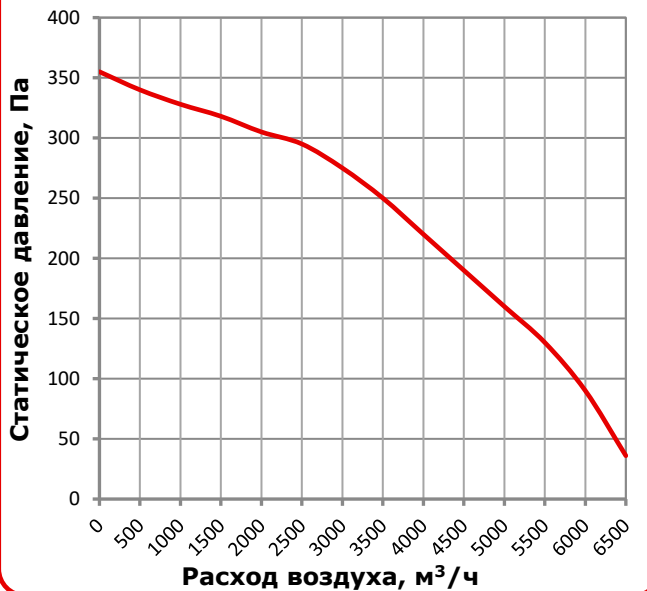
MIRAVENT VA 6000 EC
