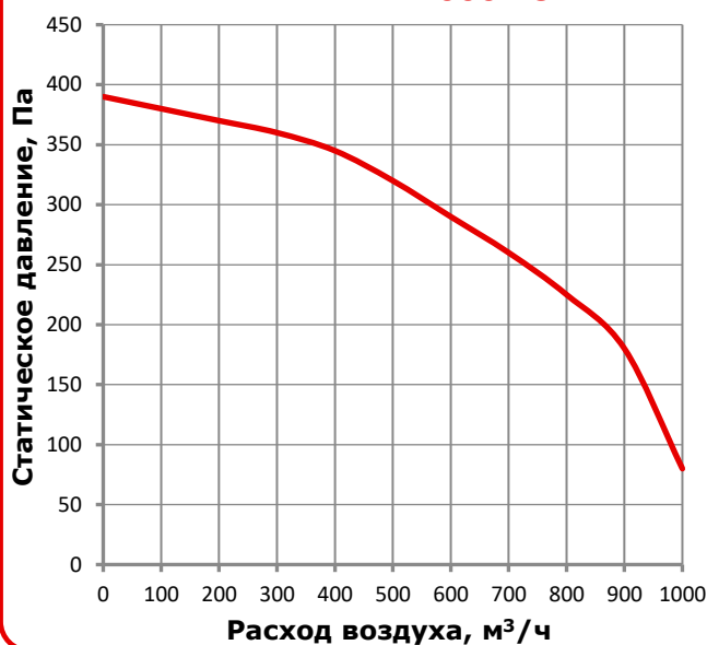
MIRAVENT VA 1000 EC
