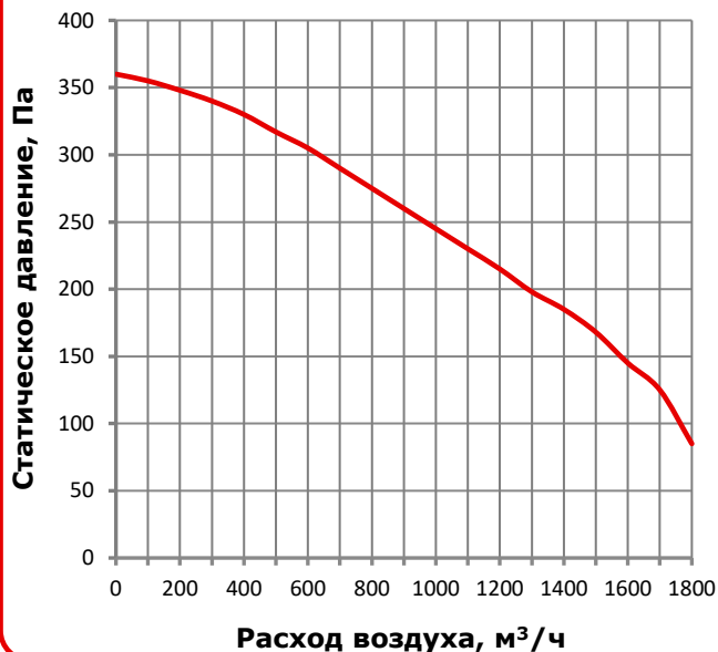
MIRAVENT VA 1600 EC
