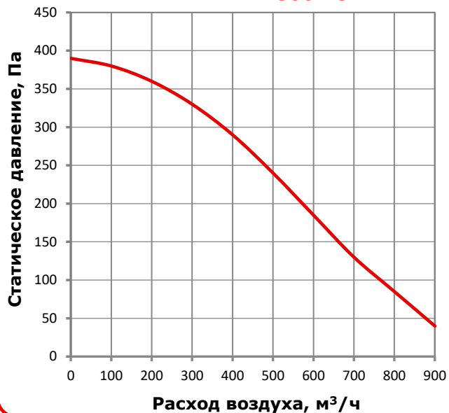
MIRAVENT VA 800 EC
