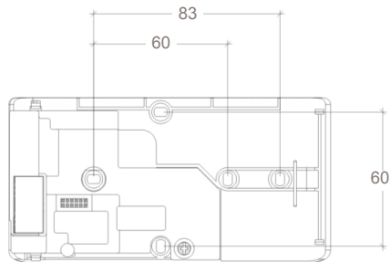
МЕЖДУОСНЫЕ РАССТОЯНИЯ ОТВЕРСТИЙ
