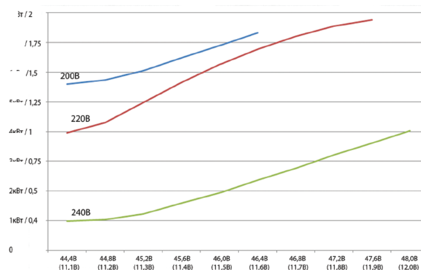
Зависимость, максимально возможной подкачки, от напряжения на АКБ.
