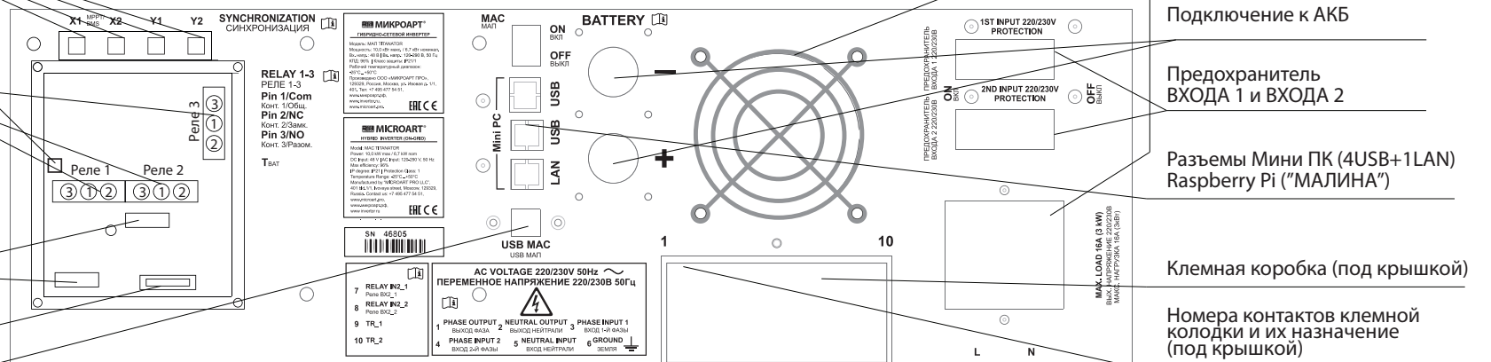
Рисунок 2.А Внешний вид инвертора (вертикальный корпус), нижняя сторона
