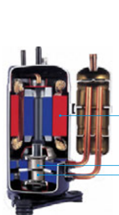
Компрессор (двухроторный)
