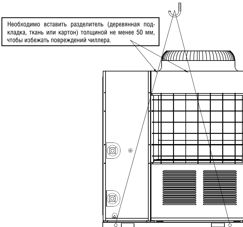
Рис. 2-1. Подъем модуля
