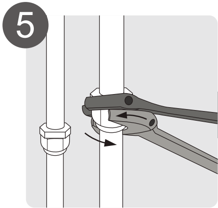
5 Соединить трубопроводы (стр.25)
