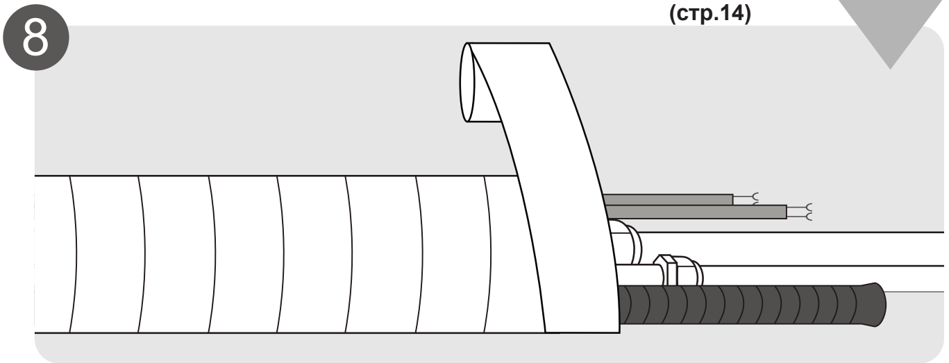
8 Обвязать трубопроводы и кабели (в некоторых районах США не нужно) (стр.18)
