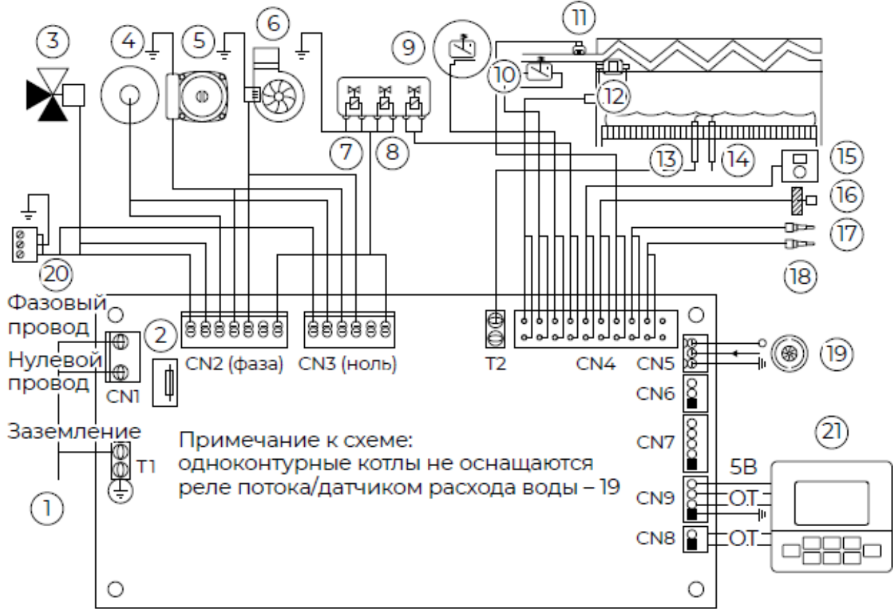
Схема котла METEOR B30 с поддержкой OpenTherm
