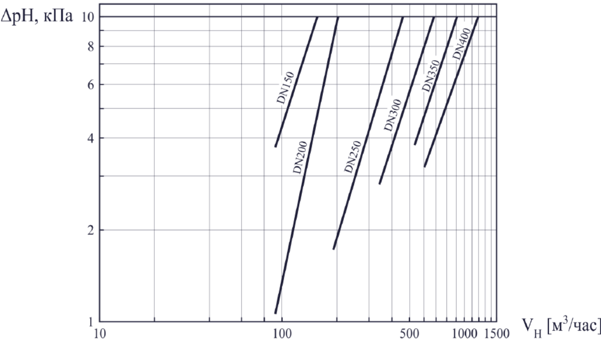
Гидравлическое сопротивление
