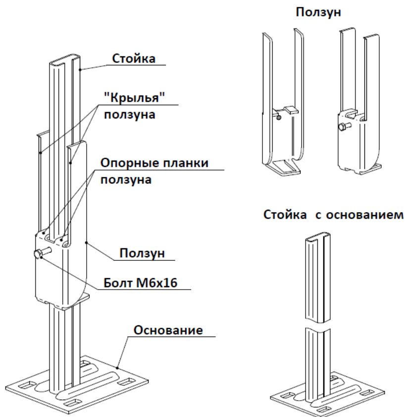
Кронштейн K11.31
