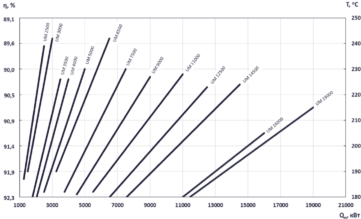
График КПД и температуры уходящих газов в зависимости от нагрузки
