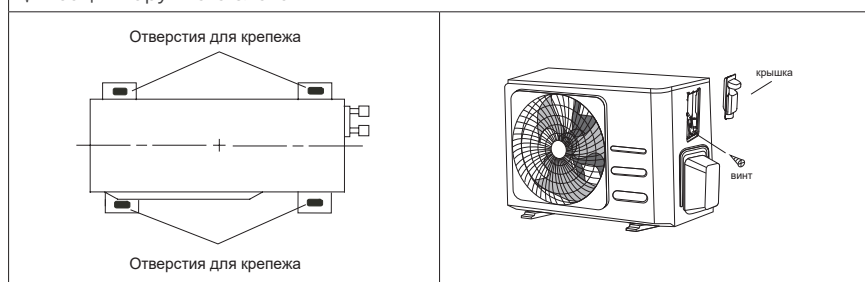
Фиксация наружного блока
