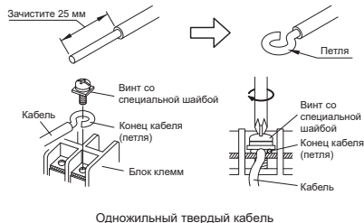
Одножильный твердый кабель
