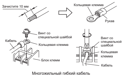
Многожильный гибкий кабель
