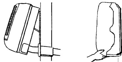
2. Панель крепления модуля может быть использована для крепления модуля в наклонном положении. (Смотрите рисунок) для облегчения проведения труб.
