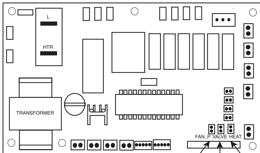
Перемычка приоритета циркулирующего воздуха Перемычка клапанного управления Перемычка теплового насоса
