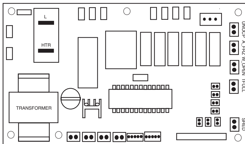
← Режим "Свободно" ← Режим "Антифриз" ← Режим "Открытое окно" ← Подключить к реле уровня ← Режим "Нагрузка"
