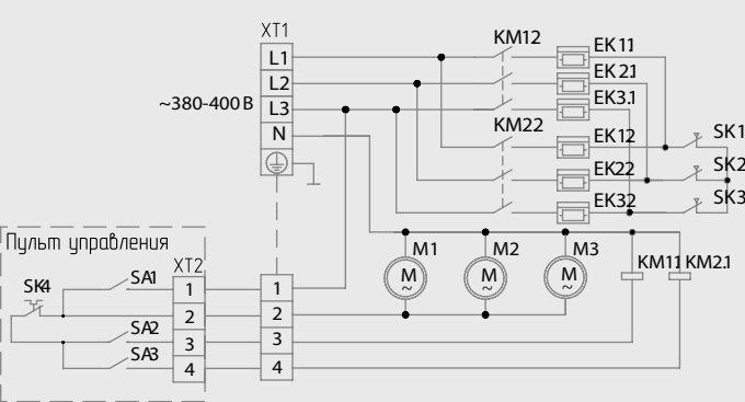
Схема электрическая модель LTZ-9.0 S
