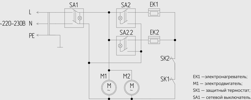
Схема электрическая LTZ-3.0 T
