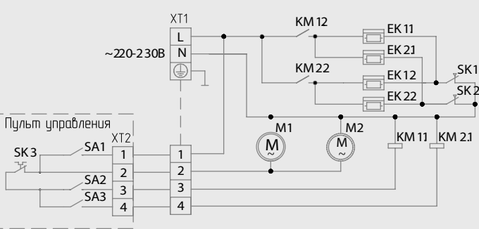
Схема электрическая модель LTZ-6.0 S
