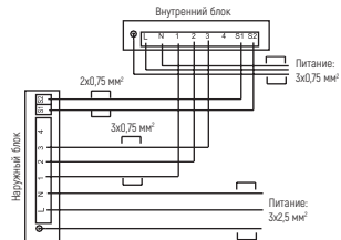
Схема соединений (Модель LAC-24TD)
