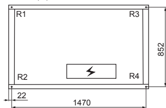
LUC-F(D)HDA30CAW
