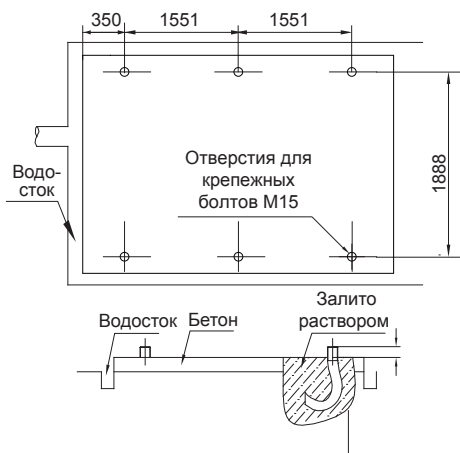
250 кВт
