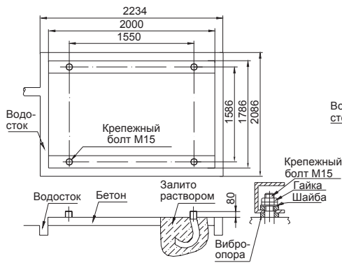
130 кВт
