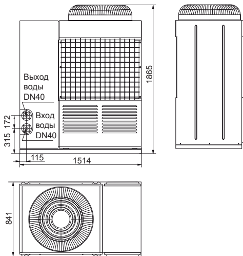
LUC-F(D)HDA30CAW
