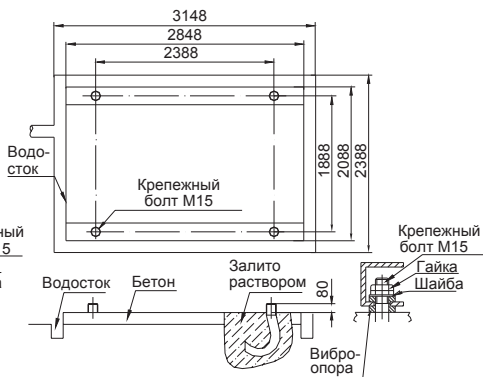
185 кВт
