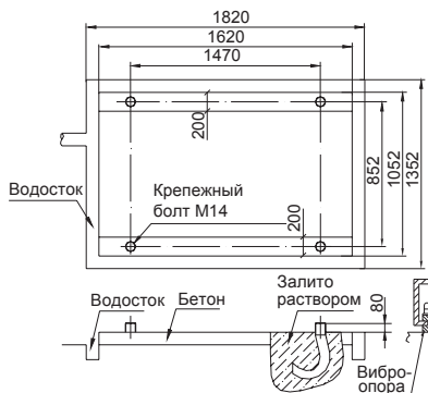
30 кВт
