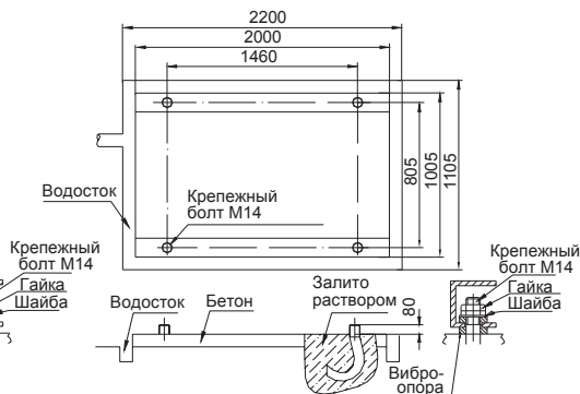
65 кВт
