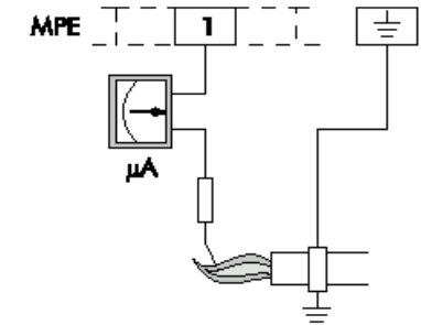
ПОДКЛЮЧЕНИЕ МИКРОАМПЕРМЕТРА
