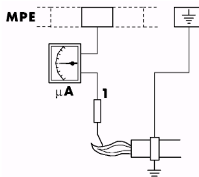
подключение микроамперметра
