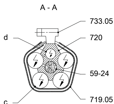
Рис. 53: Разрез А–А, расположение силового кабеля и кабеля управления, а также несущего троса
