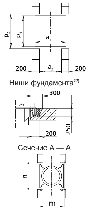
Выносной элемент X: Установочная плита шахты Вид: без насоса
