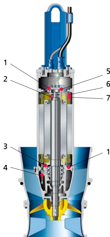
Рис. 23: Позиции датчиков
