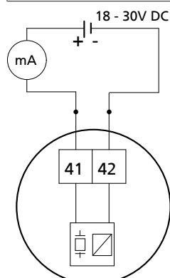
Рис. 25: Подключение вибродатчика
