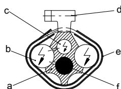
Рис. 14: Разрез кабельной укладки
