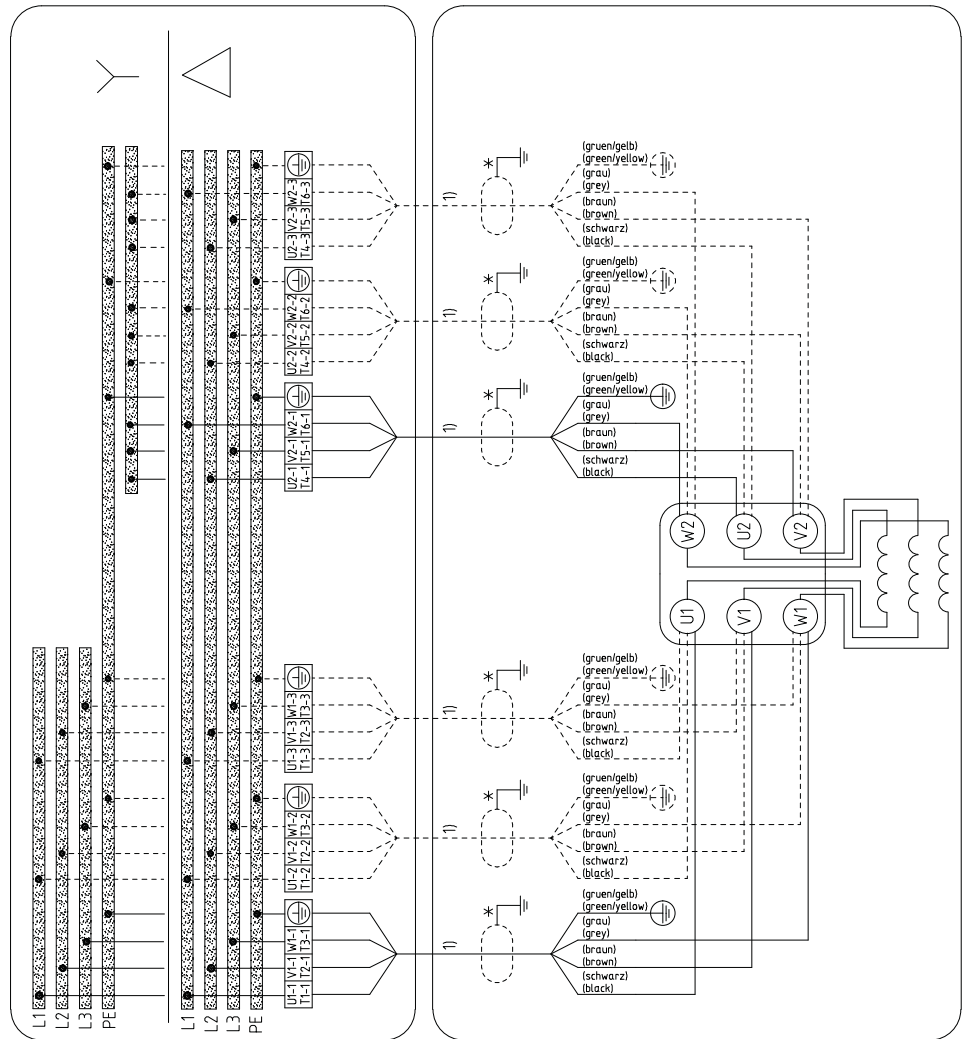
Рис. 54: Электрическая схема подключения, силовой кабель 700-470...1500-1060
