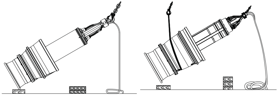
Установка насосного агрегата в вертикальное положение с помощью одного крана
