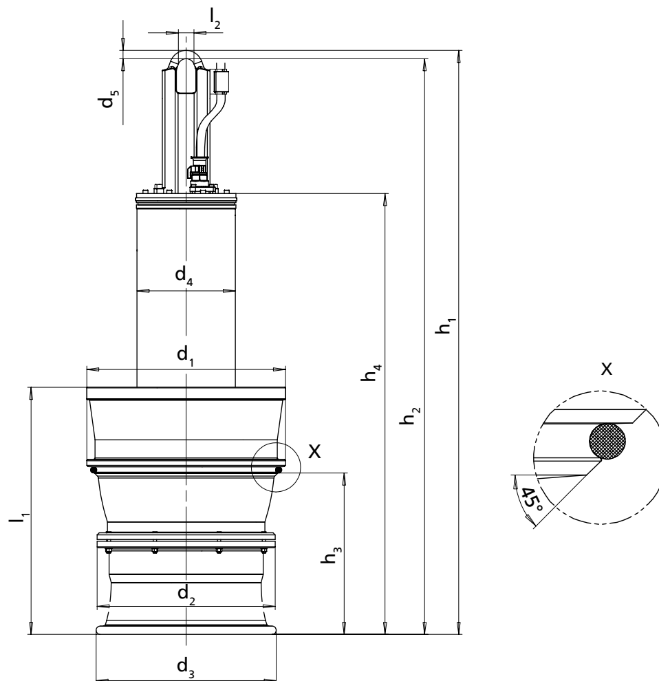
Рис. 61: Габаритный чертеж насосного агрегата
