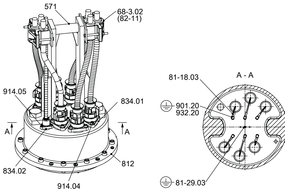
Рис. 38: Демонтаж кабеля подсоединения и кабельного ввода
