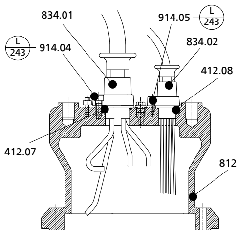
Рис. 39: Установка кабельного ввода
