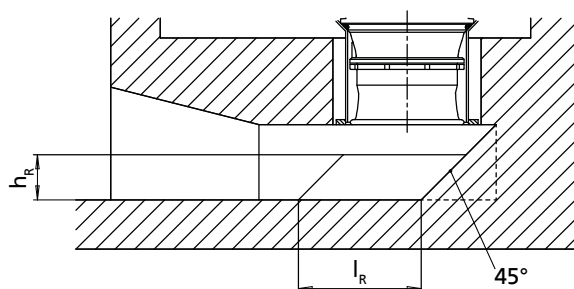
Рис. 64: Напольное ребро для закрытой камеры
