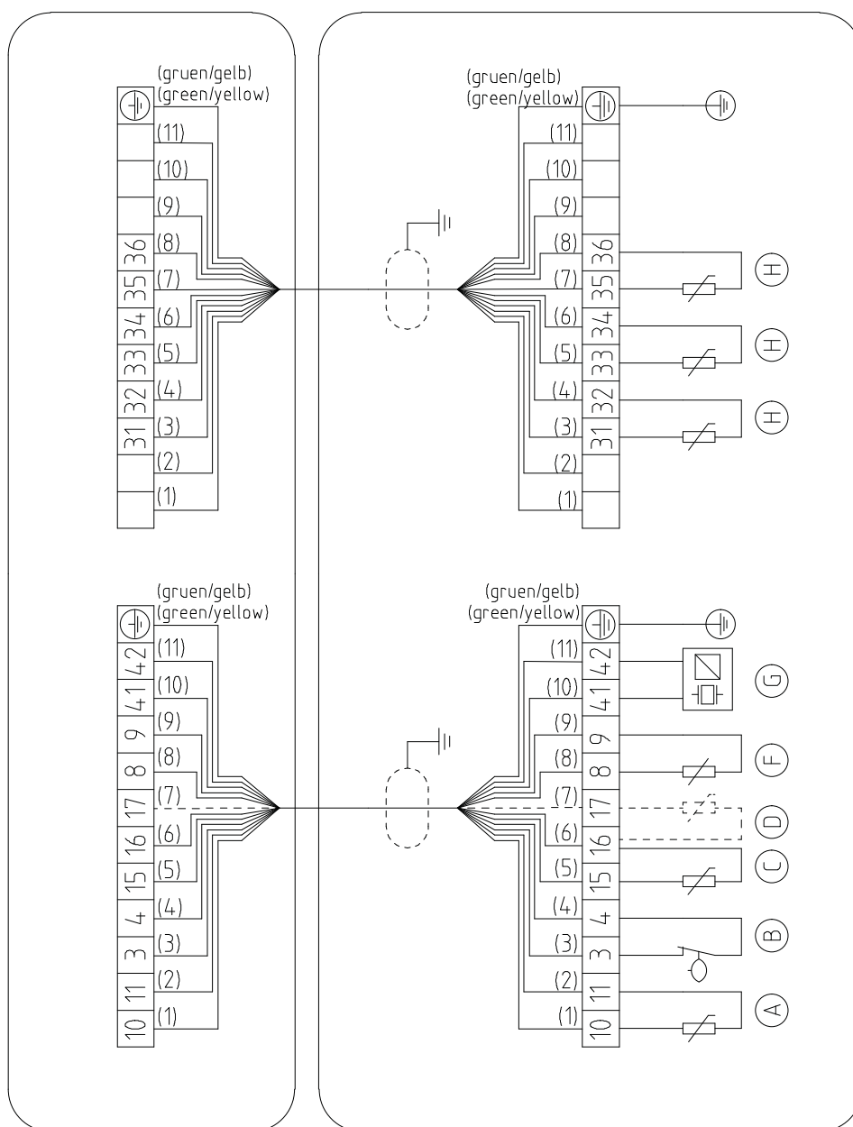
Рис. 59: Схема электрических подключений датчиков для насосных агрегатов с дополнительной системой контроля температуры двигателя Pt100 и датчиком колебаний
