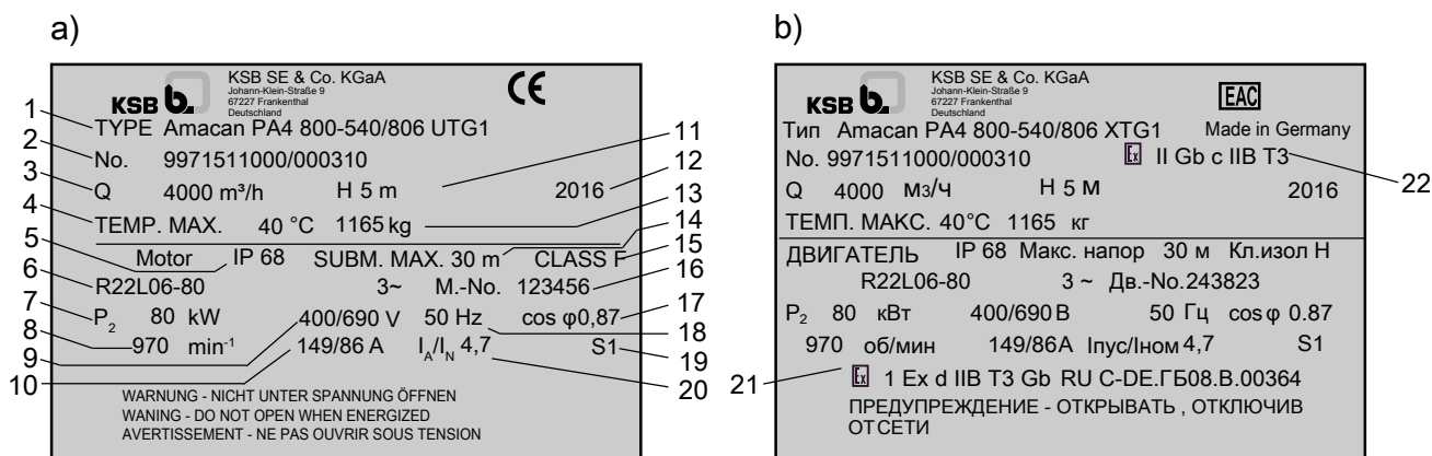
Рис. 3: Заводская табличка (пример а) без взрывозащиты б) с взрывозащитой
