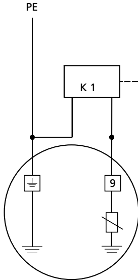
Подключение электродного реле (стандарт)
