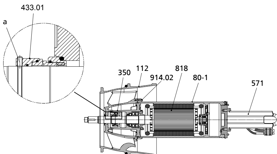
Рис. 36: Торцевое уплотнение со стороны привода
