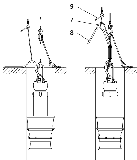
Рис. 19: Фиксация кабеля управления и силового кабеля
