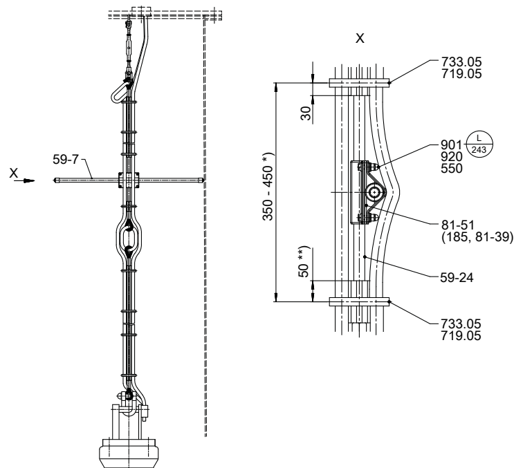
Рис. 21: Несущий трос с опорным элементом, размеры в мм
