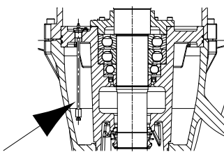
Рис. 24: Поплавковый выключатель
