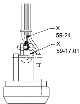
Рис. 16: X = обозначение грузоподъемности
