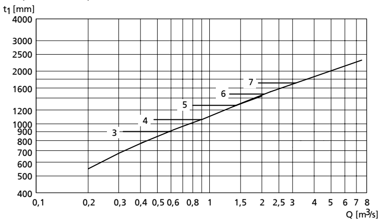
График для минимального уровня воды
