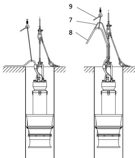
Рис. 13: Фиксация кабеля управления и силового кабеля
