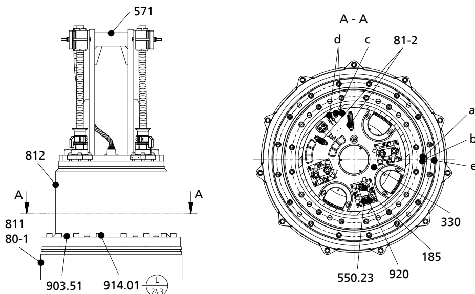
Рис. 41: Монтаж крышки корпуса двигателя
