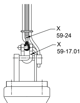
Рис. 10: X = обозначение грузоподъемности
