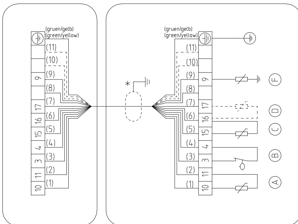
Рис. 56: Схема электрических подключений датчиков для стандартных насосных агрегатов
