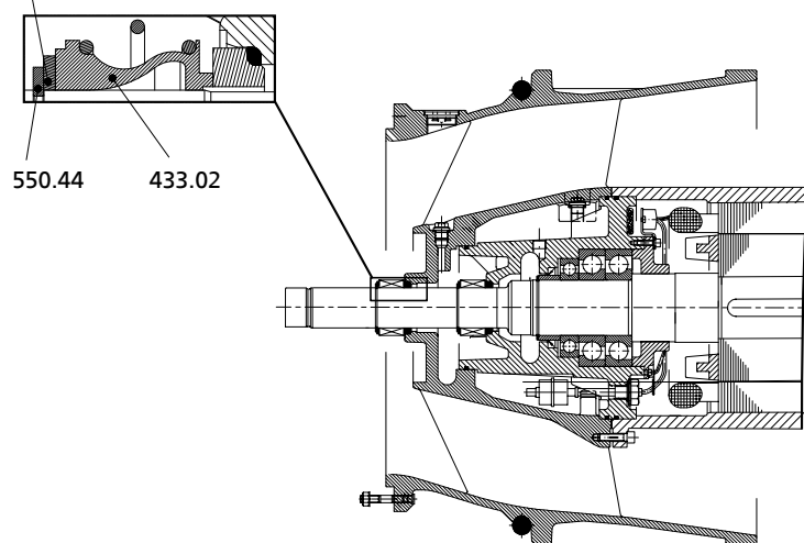
Рис. 33: Демонтаж торцевого уплотнения со стороны рабочего колеса
