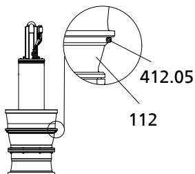
Рис. 8: Вкладывание уплотнительного кольца круглого сечения
