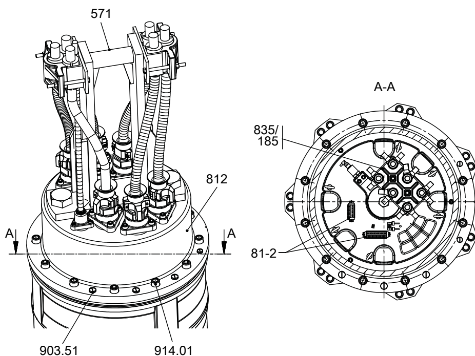
Рис. 37: Демонтаж крышки корпуса двигателя
