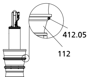
Рис. 11: Вкладывание уплотнительного кольца круглого сечения
