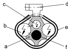
Рис. 20: Поперечное сечение кабельной сборки
