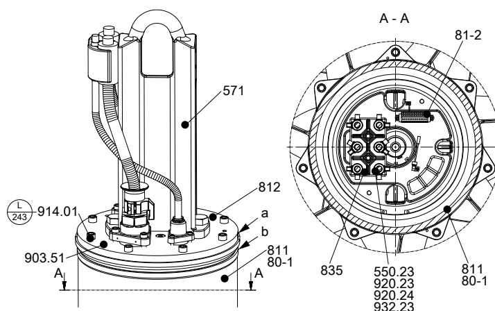
Рис. 40: Монтаж крышки корпуса двигателя
