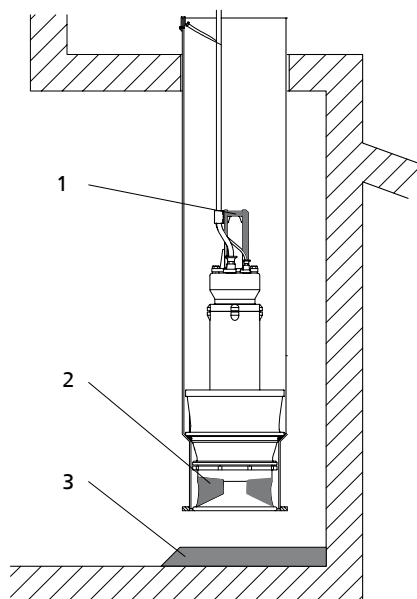
Рис. 63: Положение установки насосного агрегата
