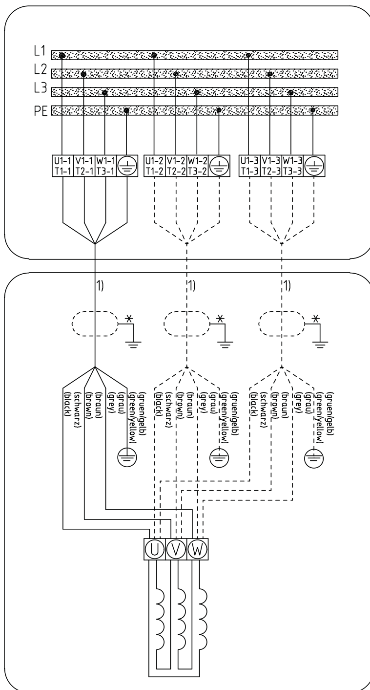
Рис. 55: Электрическая схема подключения, силовой кабель 1600-1060
