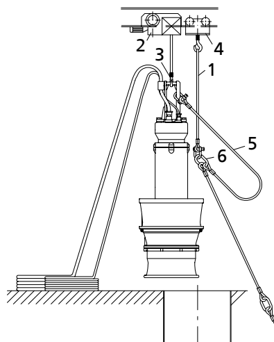
Рис. 12: Подъем и позиционирование насосного агрегата
