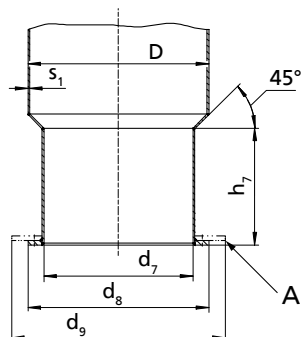
Рис. 62: Габаритный чертеж трубы-шахты
