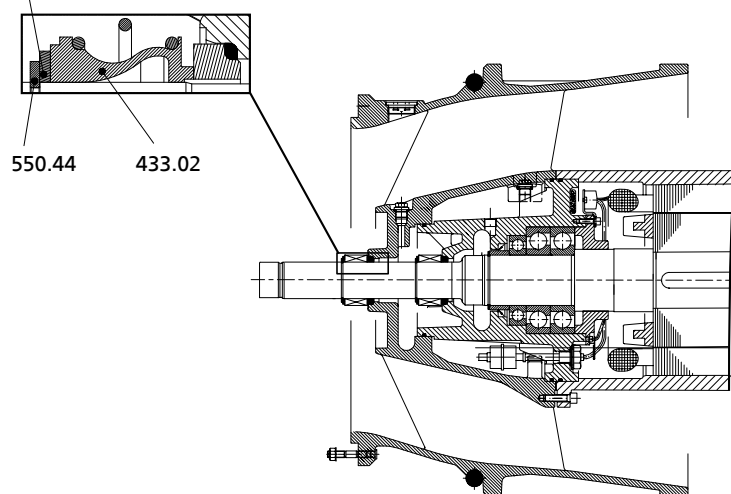
Рис. 44: Монтаж торцевого уплотнения на стороне рабочего колеса
