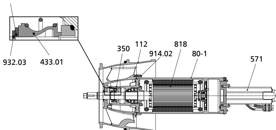
Рис. 35: Демонтаж торцевого уплотнения со стороны привода
