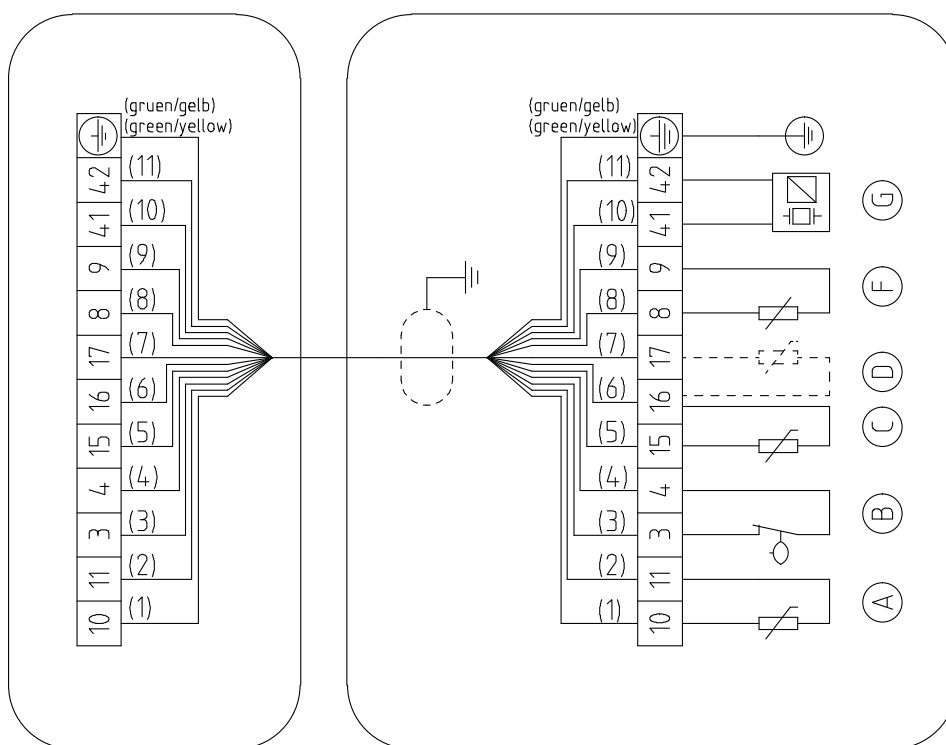
Рис. 57: Схема электрических подключений датчиков для насосных агрегатов с дополнительным контролем с помощью датчика колебаний
