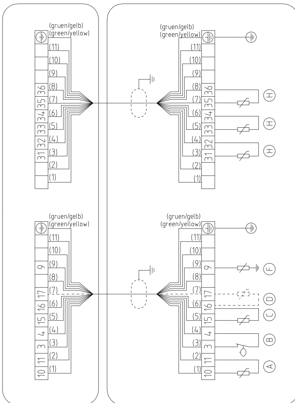
Рис. 58: Схема электрических подключений датчиков для насосных агрегатов с дополнительной системой контроля температуры двигателя Pt100
