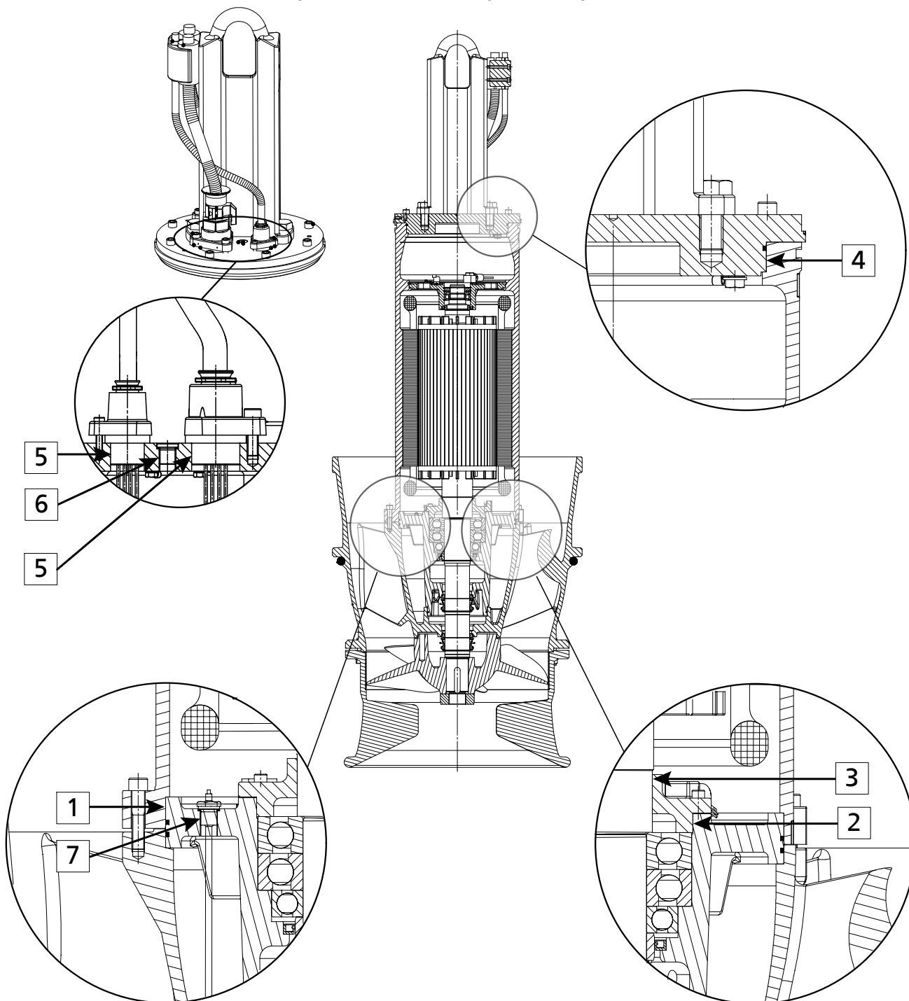
Рис. 60: Взрывозащитные зазоры для взрывозащищенных двигателей
