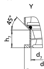
Выносной элемент Y: Опорное кольцо
