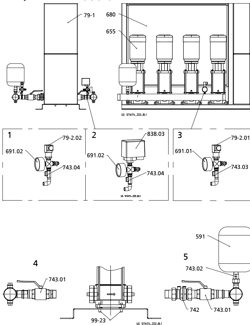
Рис. 9: Сборочный чертеж Нуамат К с Movitec 2, 4, 6, 10, 15
