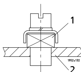
Рис. 5: Подключение провода выравнивания потенциалов
