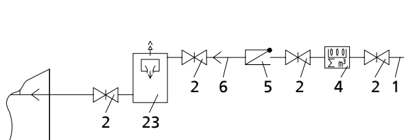
Рис. 11: Технологическая схема, непосредственное подключение - части, изображенные на сером фоне, входят в комплект поставки
