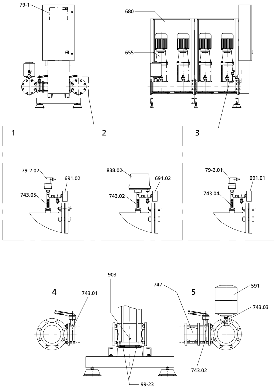
Рис. 10: Сборочный чертеж Нямат К с Movitec 25, 40, 60, 90
