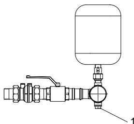
Рис. 6: Удаление воздуха из напорного резервуара и опорожнение
