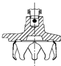
Дроссельная головка для типоразмеров, начиная с DN 125
