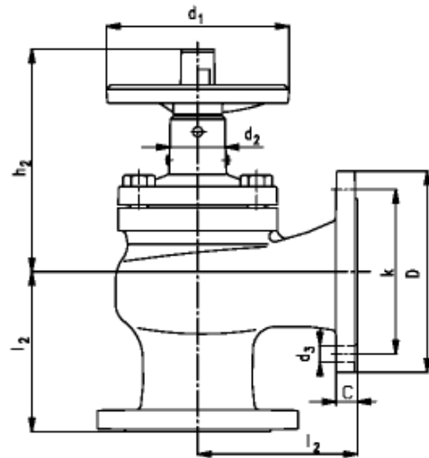
Угловая форма
