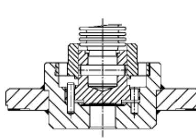
Разгрузочная головка для типоразмеров, начиная с DN 125
