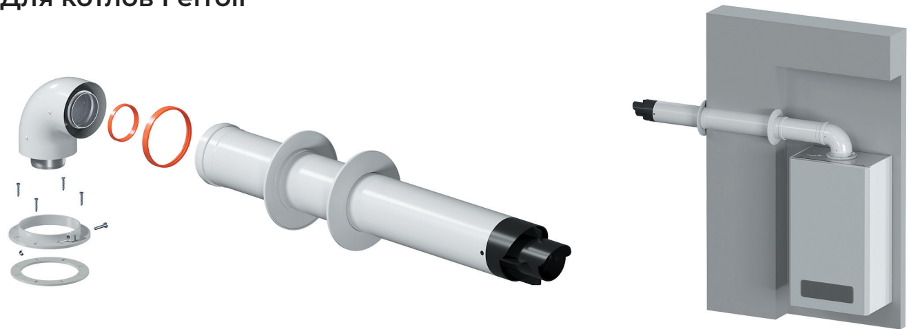
Один из вариантов присоединения к котлам. Остальные схемы смотри на стр. 163
