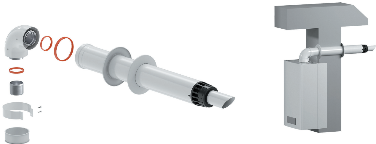
Один из вариантов присоединения к котлам. Остальные схемы смотри на стр. 163
