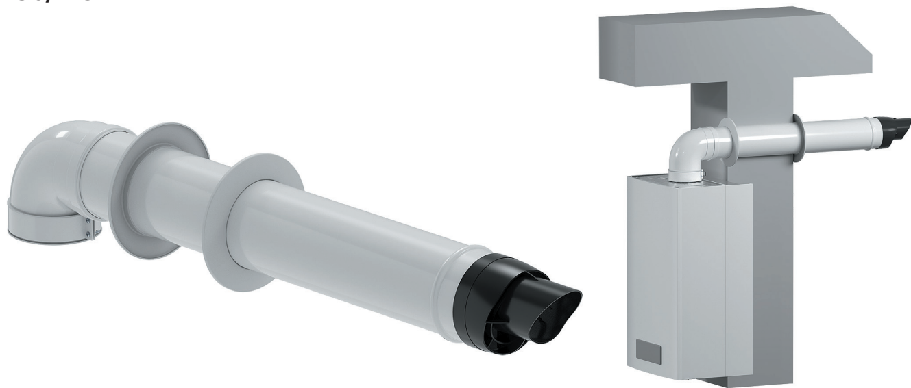
Один из вариантов присоединения к котлам. Остальные схемы смотри на стр. 163
