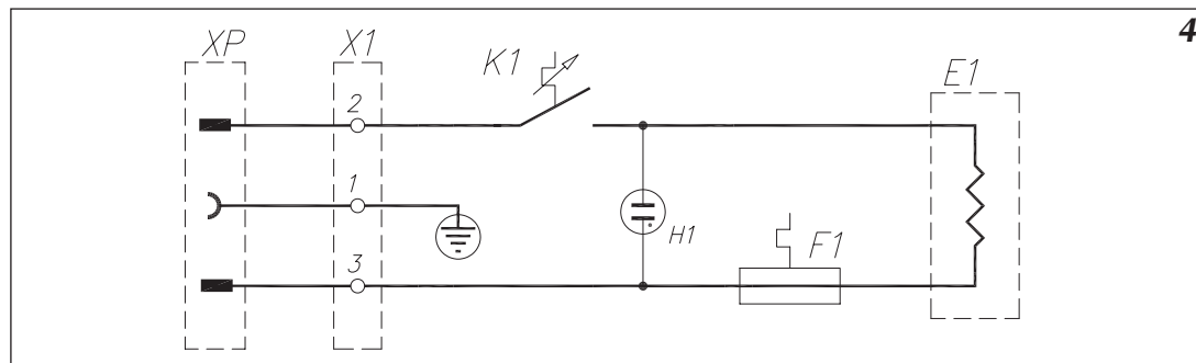
Рис.4 Принципиальная схема
