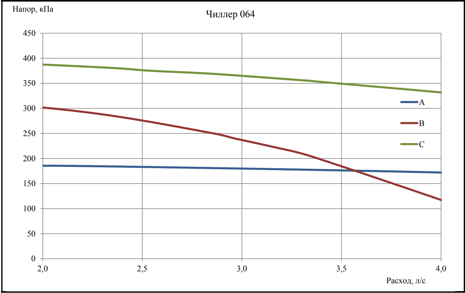
Приложение 8. Графики зависимости полного напора насосов от расхода воды.
