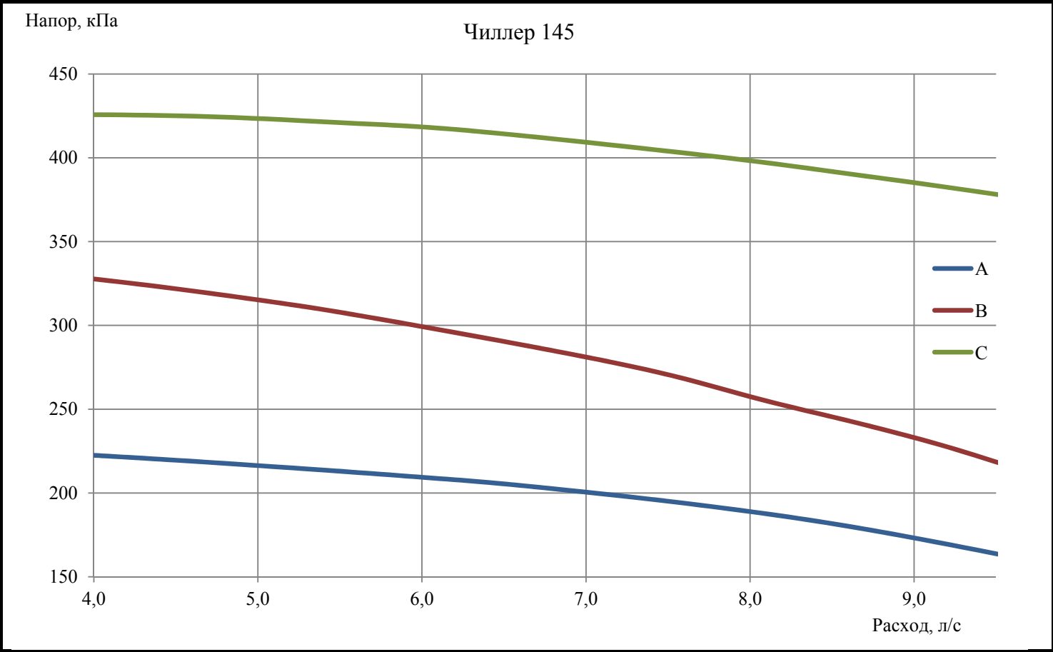
Приложение 8. Графики зависимости полного напора насосов от расхода воды.
