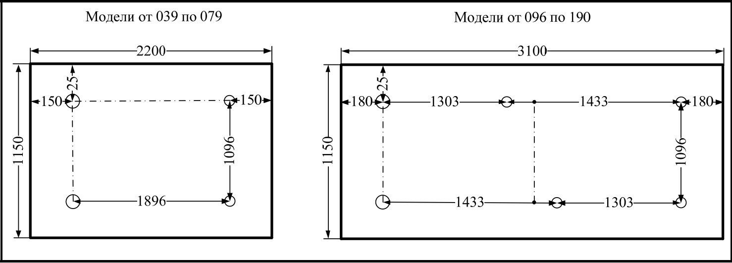
Рисунок 1.8.1. Схема крепления виброизоляторов к чиллеру (вид сверху).
