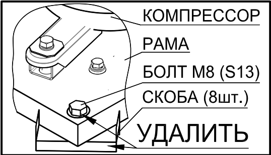
Рисунок 1.8.2. Транспортировочные скобы.
