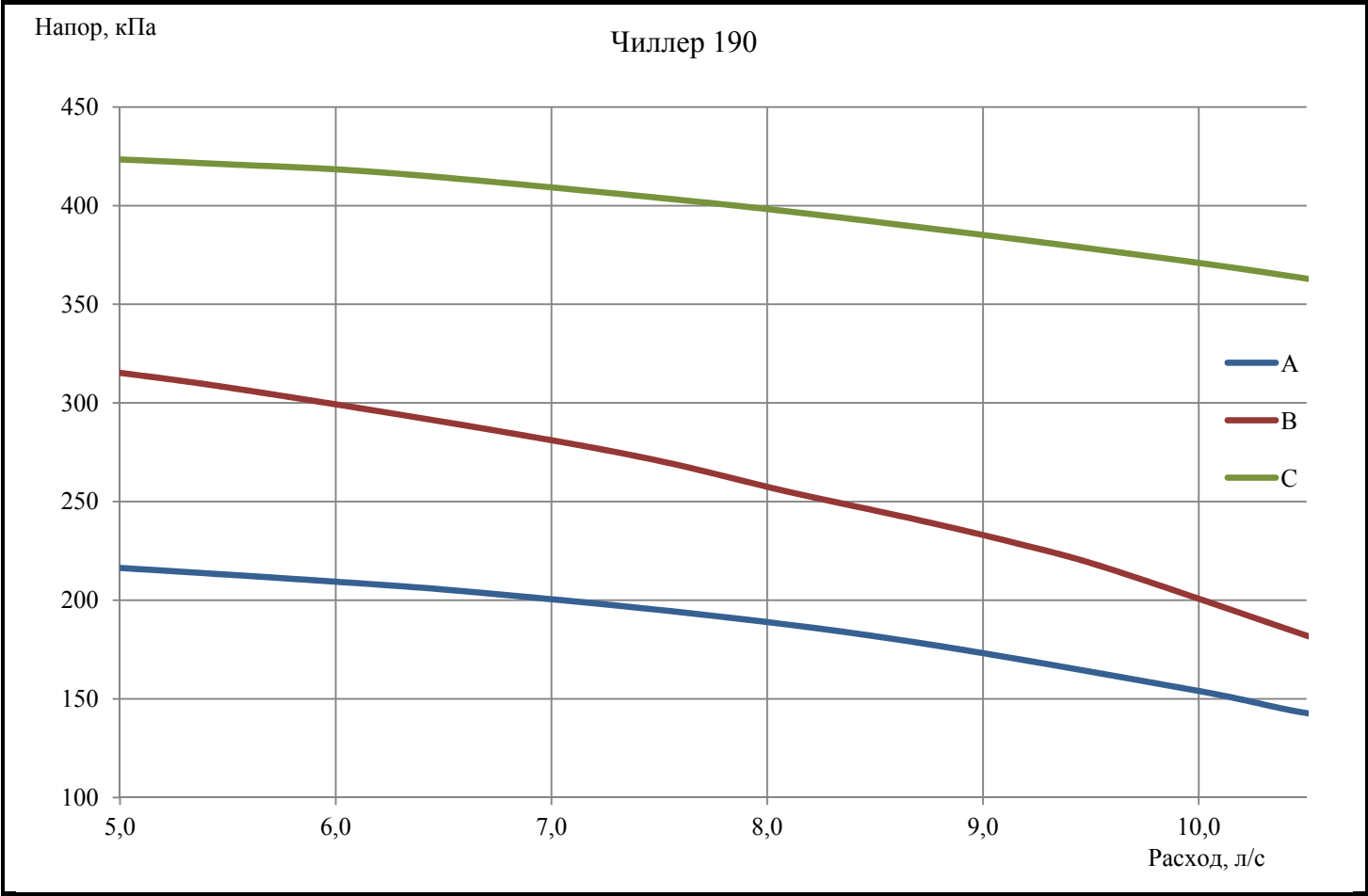
Приложение 8. Графики зависимости полного напора насосов от расхода воды.
