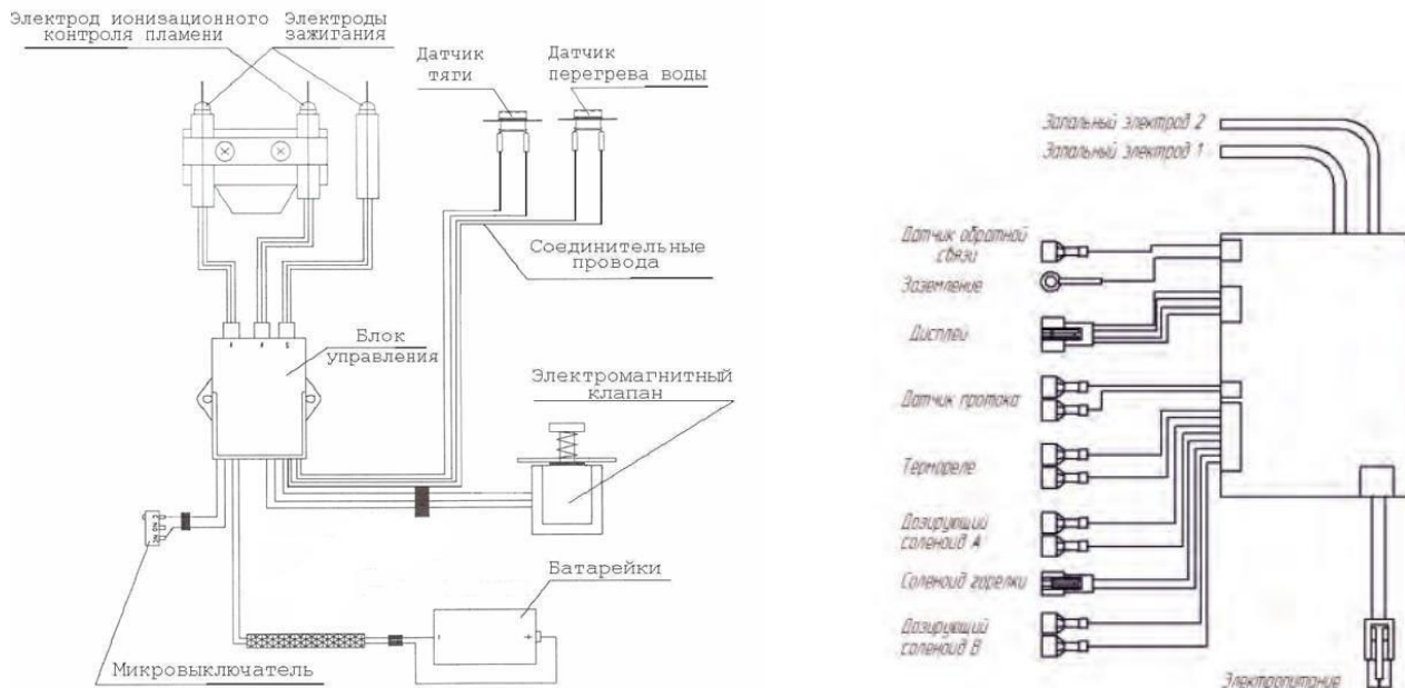
Рис. 2. Схема электрическая
