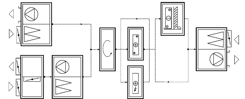
Возможное подключение секций
