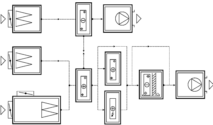
Возможное подключение секций
