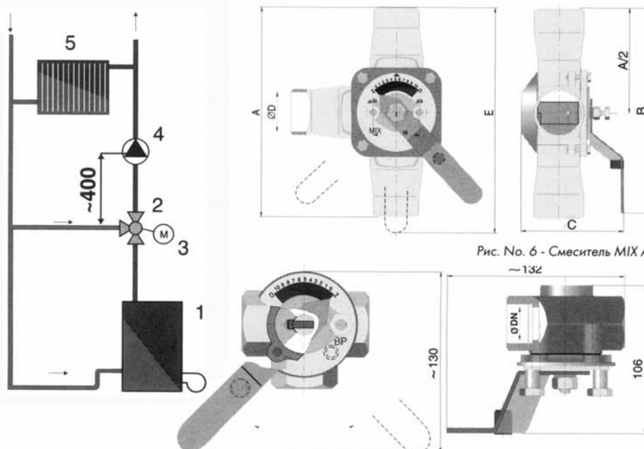
Рис. No. 5 - Смеситель MIX BP
