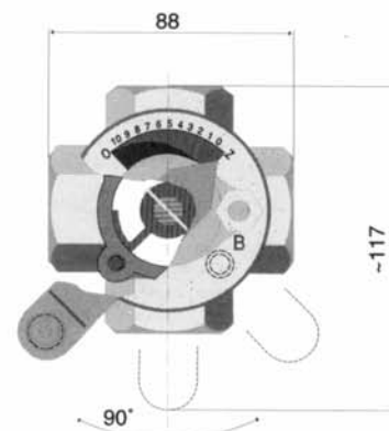
Рис. No. 3 - Смеситель DUOMIX B
