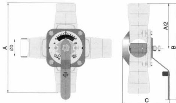
Рис. No. 1: DUOMIX AO - размерный чертеж + таблица
