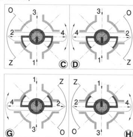
Рис. No. 7 - Возможности подключения смесителей DUOMIX.
