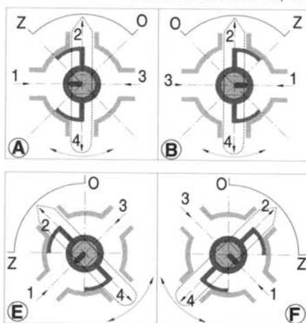
Рис. No. 8: возможности подключения смесителей MIX.
