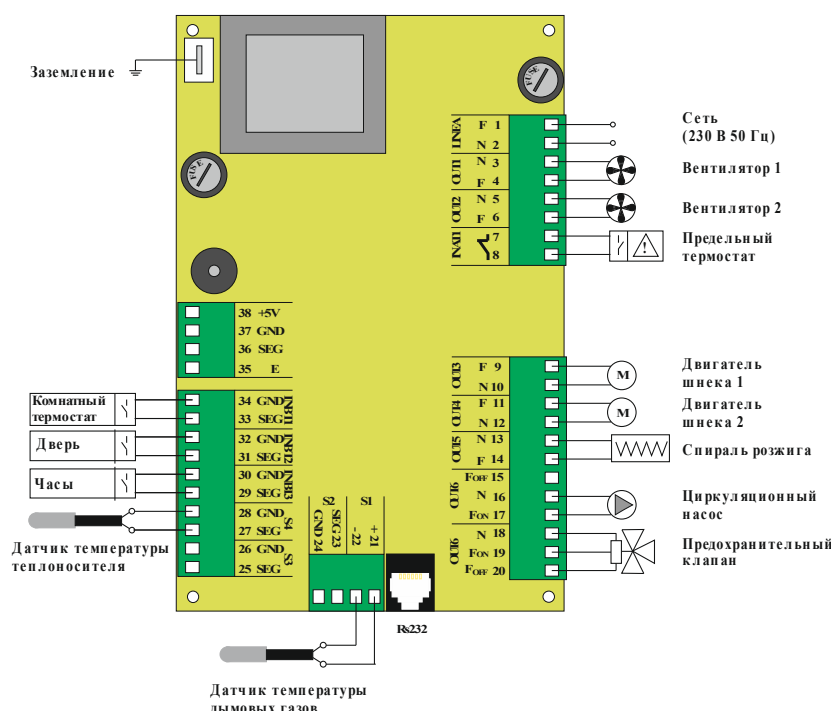
Рис. 2 Схема подключения входов и выходов программируемого контроллера.
