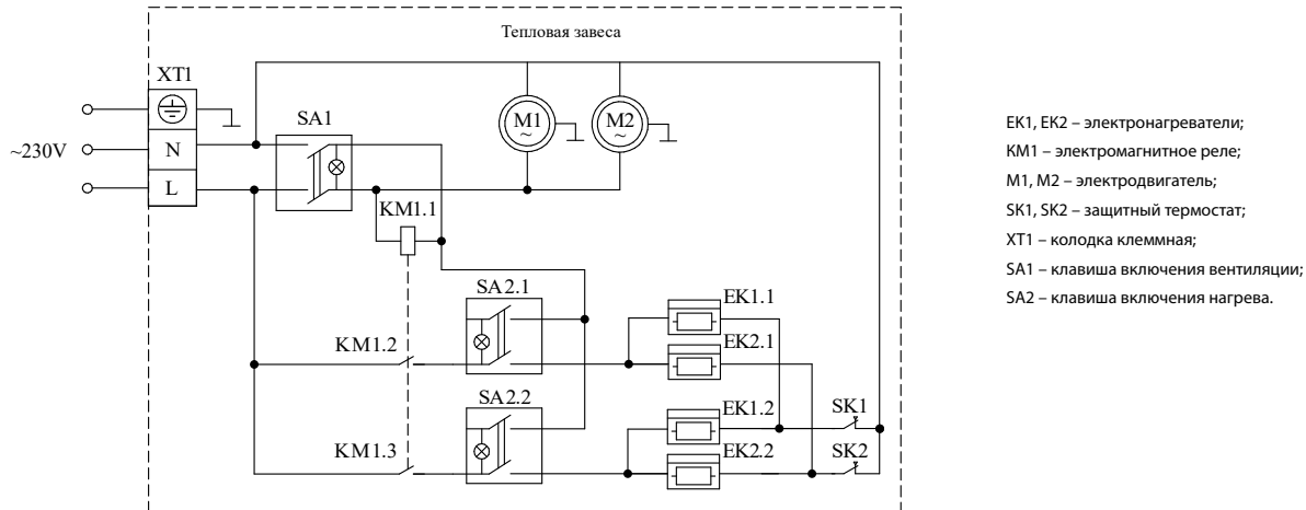
СХЕМА ЭЛЕКТРИЧЕСКАЯ ПРИНЦИПИАЛЬНАЯ ПОДКЛЮЧЕНИЯ ЗАВЕСЫ KVC-A08E5-11
