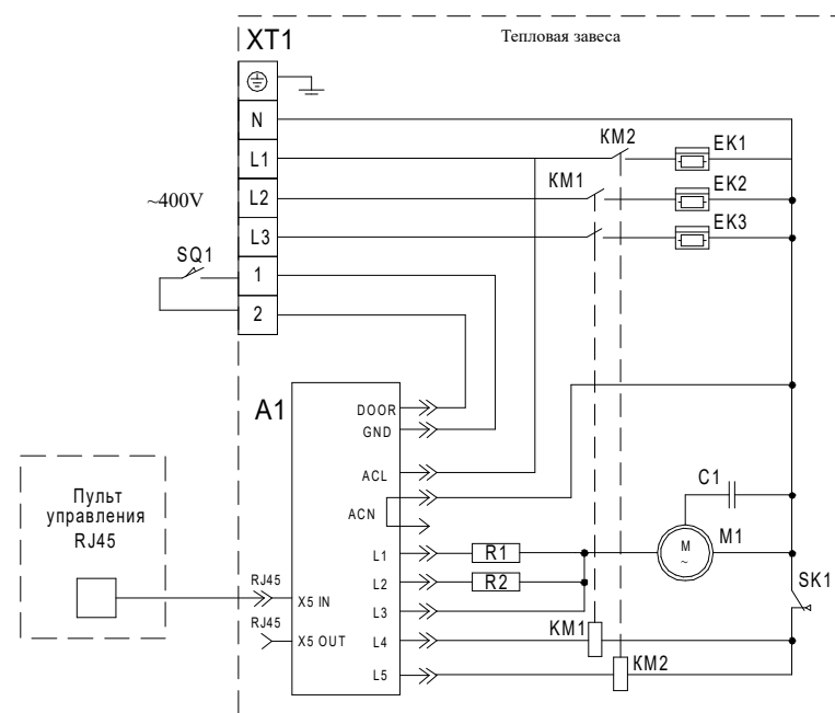
СХЕМА ЭЛЕКТРИЧЕСКАЯ ПРИНЦИПИАЛЬНАЯ ПОДКЛЮЧЕНИЯ ЗАВЕС KVC-B10E09-31, KVC-B10E09-32, KVC-B15E09-31, KVC-B15E09-32, KVC-B15E12-31, KVC-B15E12-32 К ПУЛЬТУ УПРАВЛЕНИЯ KRC-11
