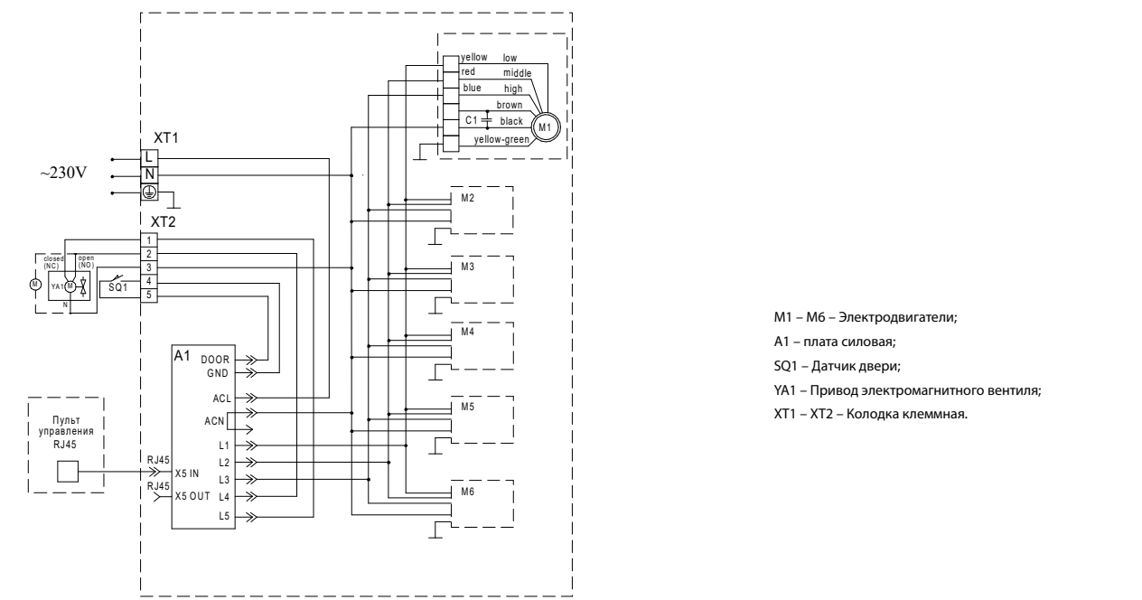
СХЕМА ЭЛЕКТРИЧЕСКАЯ ПРИНЦИПИАЛЬНАЯ ПОДКЛЮЧЕНИЯ ЗАВЕС KVC-S25W45-31 MT, KVC-S25W45-31 GL, KVC-S25W45-31 SL К ПУЛЬТУ УПРАВЛЕНИЯ KRC-12
