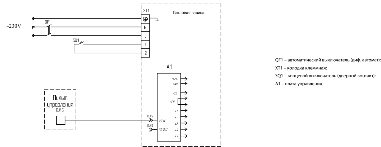
СХЕМА ЭЛЕКТРИЧЕСКАЯ ПРИНЦИПИАЛЬНАЯ ПОДКЛЮЧЕНИЯ ПУЛЬТА KRC-14
