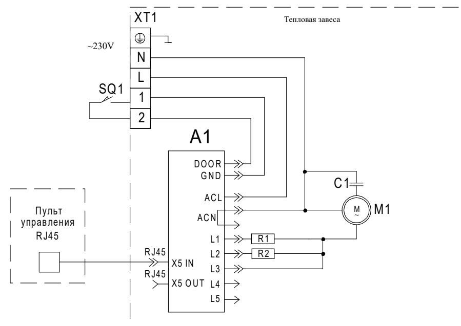
СХЕМА ЭЛЕКТРИЧЕСКАЯ ПРИНЦИПИАЛЬНАЯ ПОДКЛЮЧЕНИЯ ЗАВЕС KVC-B10V-11 И KVC-B15V-11 К ПУЛЬТУ УПРАВЛЕНИЯ KRC-14
