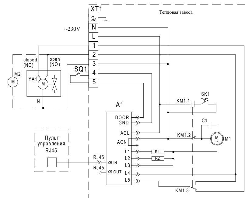
СХЕМА ЭЛЕКТРИЧЕСКАЯ ПРИНЦИПИАЛЬНАЯ ПОДКЛЮЧЕНИЯ ЗАВЕС KVC-B10W8-11, KVC-B15W14-11 К ПУЛЬТУ УПРАВЛЕНИЯ KRC-12
