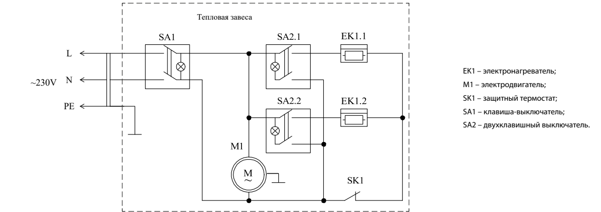
СХЕМА ЭЛЕКТРИЧЕСКАЯ ПРИНЦИПИАЛЬНАЯ ПОДКЛЮЧЕНИЯ ЗАВЕСЫ KVC-A06E3-11
