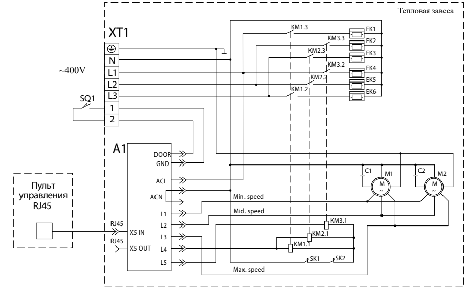
СХЕМА ЭЛЕКТРИЧЕСКАЯ ПРИНЦИПИАЛЬНАЯ ПОДКЛЮЧЕНИЯ ЗАВЕС KVC-P15E12-33 К ПУЛЬТУ УПРАВЛЕНИЯ KRC-11
