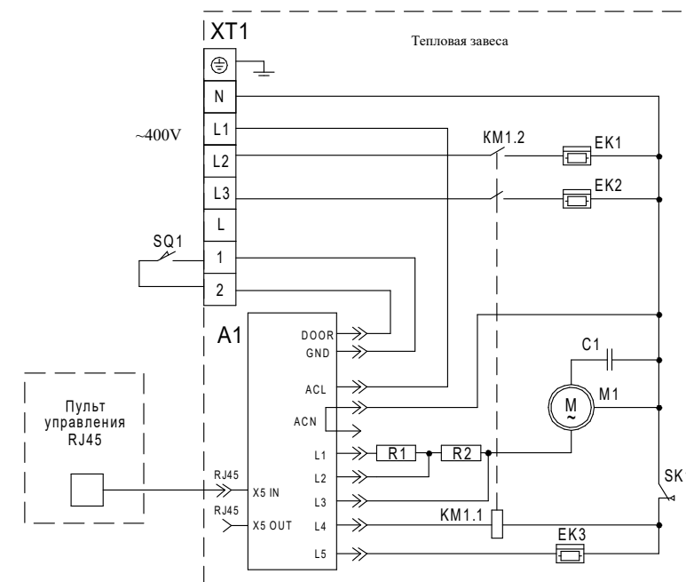
СХЕМА ЭЛЕКТРИЧЕСКАЯ ПРИНЦИПИАЛЬНАЯ ПОДКЛЮЧЕНИЯ ЗАВЕС KVC-C10E6-01, KVC-C15E6-01 К ПУЛЬТУ УПРАВЛЕНИЯ KRC-11
