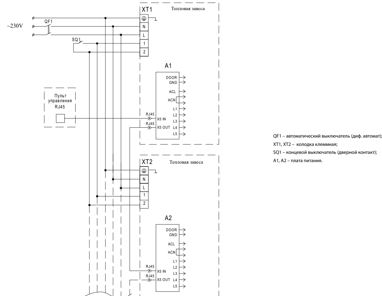
СХЕМА ЭЛЕКТРИЧЕСКАЯ ПРИНЦИПИАЛЬНАЯ ГРУППОВОГО ПОДКЛЮЧЕНИЯ ЗАВЕС К ОДНОМУ ПУЛЬТУ УПРАВЛЕНИЯ KRC-14
