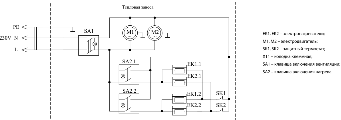
СХЕМА ЭЛЕКТРИЧЕСКАЯ ПРИНЦИПИАЛЬНАЯ ПОДКЛЮЧЕНИЯ ЗАВЕСЫ KVC-A08E3-11
