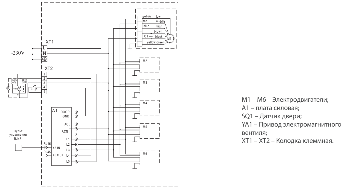
СХЕМА ЭЛЕКТРИЧЕСКАЯ ПРИНЦИПИАЛЬНАЯ ПОДКЛЮЧЕНИЯ ЗАВЕС KVC-S25W45-31 MT, KVC-S25W45-31 GL, KVC-S25W45-31 SL К ПУЛЬТУ УПРАВЛЕНИЯ KRC-12
