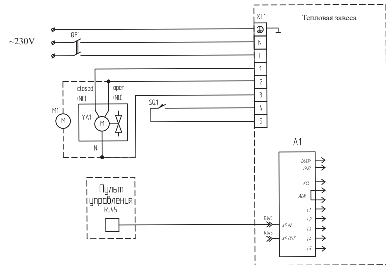
СХЕМА ЭЛЕКТРИЧЕСКАЯ ПРИНЦИПИАЛЬНАЯ ПОДКЛЮЧЕНИЯ ПУЛЬТА KRC-12
