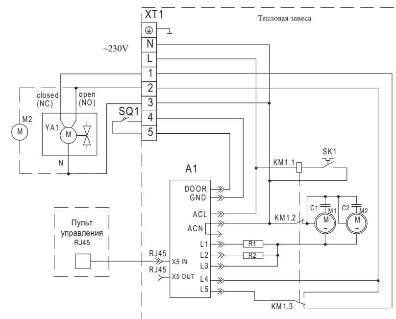
СХЕМА ЭЛЕКТРИЧЕСКАЯ ПРИНЦИПИАЛЬНАЯ ПОДКЛЮЧЕНИЯ ЗАВЕСЫ KVC-D20W50-11 К ПУЛЬТУ УПРАВЛЕНИЯ KRC-12
