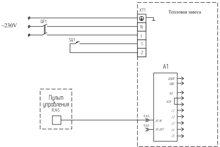
СХЕМА ЭЛЕКТРИЧЕСКАЯ ПРИНЦИПИАЛЬНАЯ ПОДКЛЮЧЕНИЯ ПУЛЬТА KRC-14
