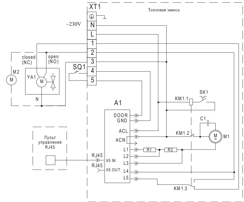
СХЕМА ЭЛЕКТРИЧЕСКАЯ ПРИНЦИПАЛЬНАЯ ПОДКЛЮЧЕНИЯ ЗАВЕС KVC-C10W12-11, KVC-C15W20-11, KVC-C20W30-11 К ПУЛЬТУ УПРАВЛЕНИЯ KRC-12
