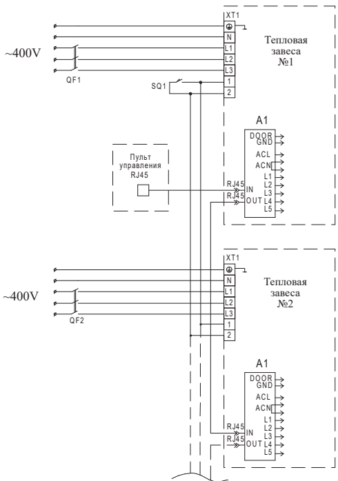
СХЕМА ЭЛЕКТРИЧЕСКАЯ ПРИНЦИПИАЛЬНАЯ ГРУППОВОГО ПОДКЛЮЧЕНИЯ ЗАВЕС KVCS20E18-31 MT, KVC-S20E18-31 GL, KVC-S20E18-31 SL, KVC-S22E18-31 MT, KVC-S22E18-31 GL, KVC-S22E18-31 SL, KVC-S25E24-31 MT, KVC-S25E24-31 GL, KVC-S25E24-31 SL С ПУЛЬТОМ УПРАВЛЕНИЯ KRC-11
