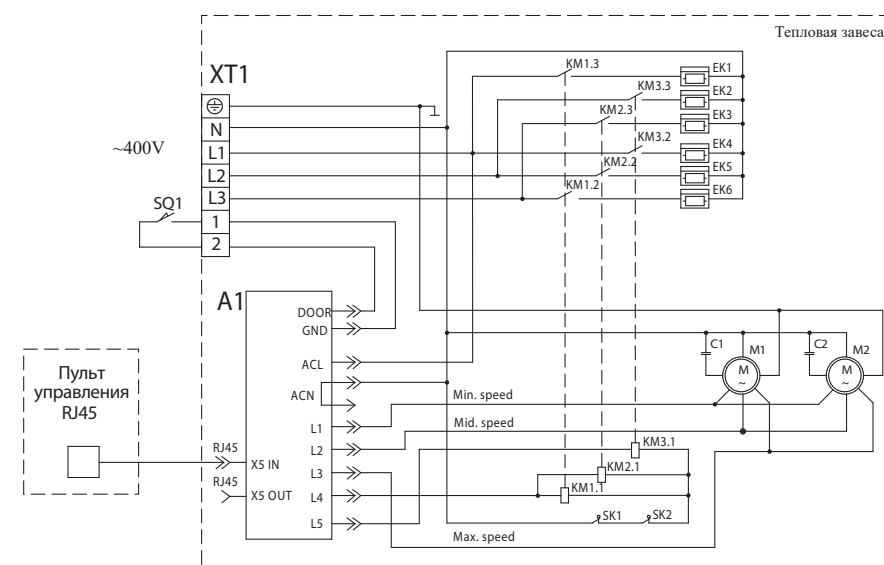
СХЕМА ЭЛЕКТРИЧЕСКАЯ ПРИНЦИПИАЛЬНАЯ ПОДКЛЮЧЕНИЯ ЗАВЕС KVC-P15E12-33 К ПУЛЬТУ УПРАВЛЕНИЯ KRC-11
