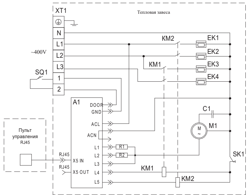
СХЕМА ЭЛЕКТРИЧЕСКАЯ ПРИНЦИПАЛЬНАЯ ПОДКЛЮЧЕНИЯ ЗАВЕС KVC-D10E12-31, KVC-D10E12-32 К ПУЛЬТУ УПРАВЛЕНИЯ KRC-11
