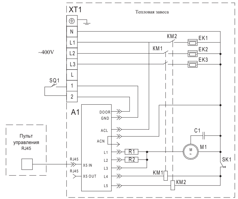
СХЕМА ЭЛЕКТРИЧЕСКАЯ ПРИНЦИПАЛЬНАЯ ПОДКЛЮЧЕНИЯ ЗАВЕС KVC-D10E9-31, KVC-D10E9-32 К ПУЛЬТУ УПРАВЛЕНИЯ KRC-11
