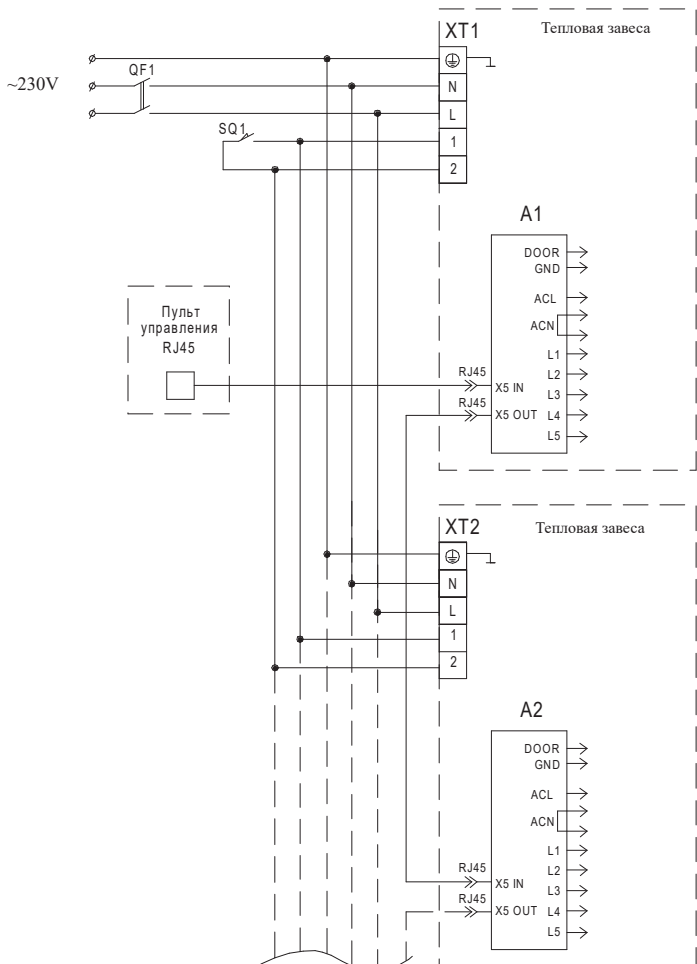
СХЕМА ЭЛЕКТРИЧЕСКАЯ ПРИНЦИПИАЛЬНАЯ ГРУППОВОГО ПОДКЛЮЧЕНИЯ ЗАВЕС К ОДНОМУ ПУЛЬТУ УПРАВЛЕНИЯ KRC-14
