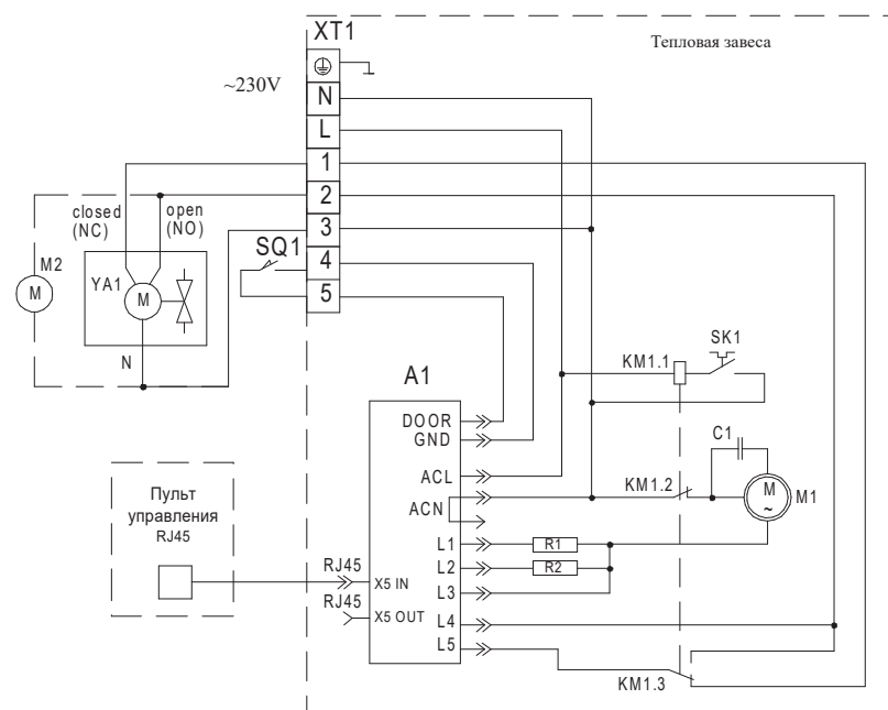
СХЕМА ЭЛЕКТРИЧЕСКАЯ ПРИНЦИПИАЛЬНАЯ ПОДКЛЮЧЕНИЯ ЗАВЕСЫ KVC-D10W20-11, KVC-D15W33-11 К ПУЛЬТУ УПРАВЛЕНИЯ KRC-12
