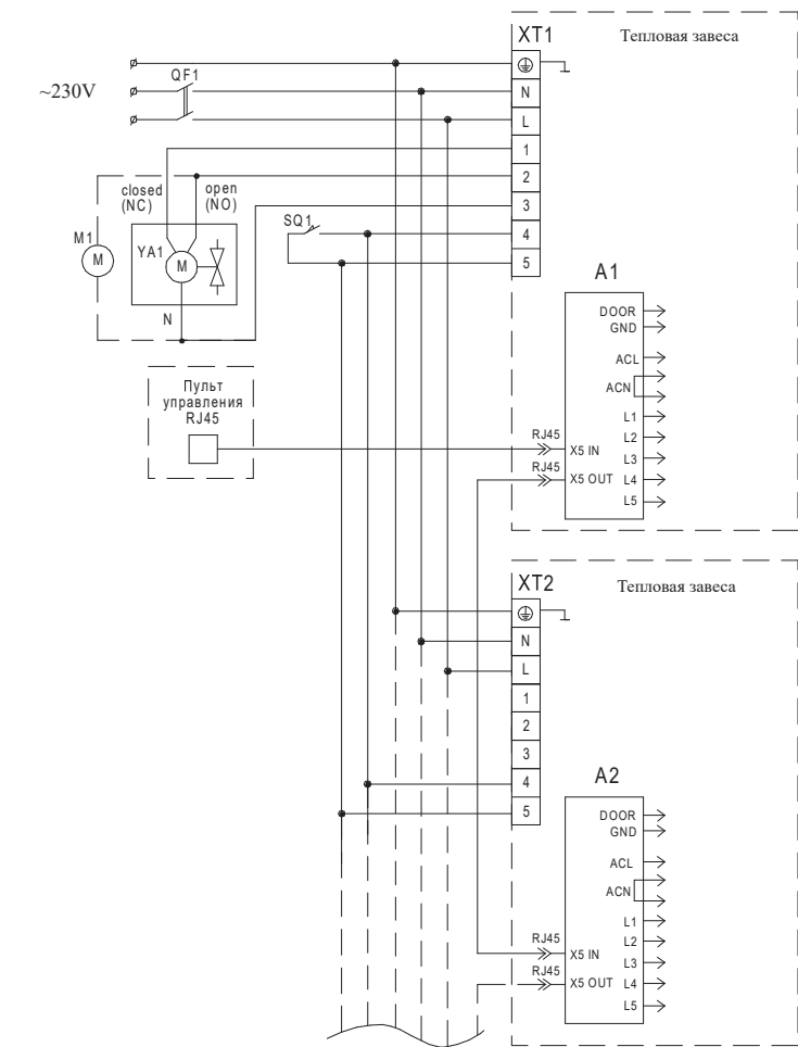
СХЕМА ЭЛЕКТРИЧЕСКАЯ ПРИНЦИПИАЛЬНАЯ ГРУППОВОГО ПОДКЛЮЧЕНИЯ ЗАВЕС К ПУЛЬТУ УПРАВЛЕНИЯ KRC-12
