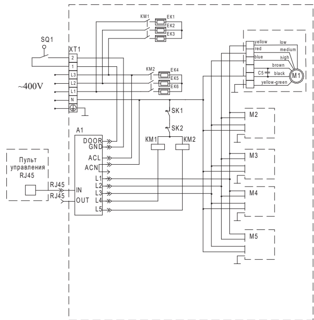
СХЕМА ЭЛЕКТРИЧЕСКАЯ ПРИНЦИПИАЛЬНАЯ ПОДКЛЮЧЕНИЯ ЗАВЕС KVC-S20E18-31 MT, KVC-S20E18-31 GL, KVC-S20E18-31 SL, KVC-S22E18-31 MT, KVC-S22E18-31 GL, KVC-S22E18-31 SL К ПУЛЬТУ УПРАВЛЕНИЯ KRC-11
