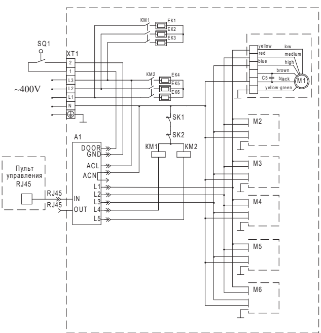
СХЕМА ЭЛЕКТРИЧЕСКАЯ ПРИНЦИПИАЛЬНАЯ ПОДКЛЮЧЕНИЯ ЗАВЕС KVC-S25E24-31 MT, KVC-S25E24-31 GL, KVC-S25E24-31 SL К ПУЛЬТУ УПРАВЛЕНИЯ KRC-11
