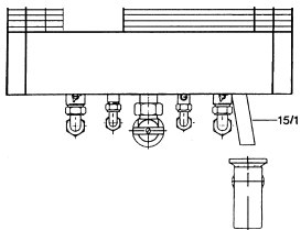
Рис. 11 15/1 - труба слива
