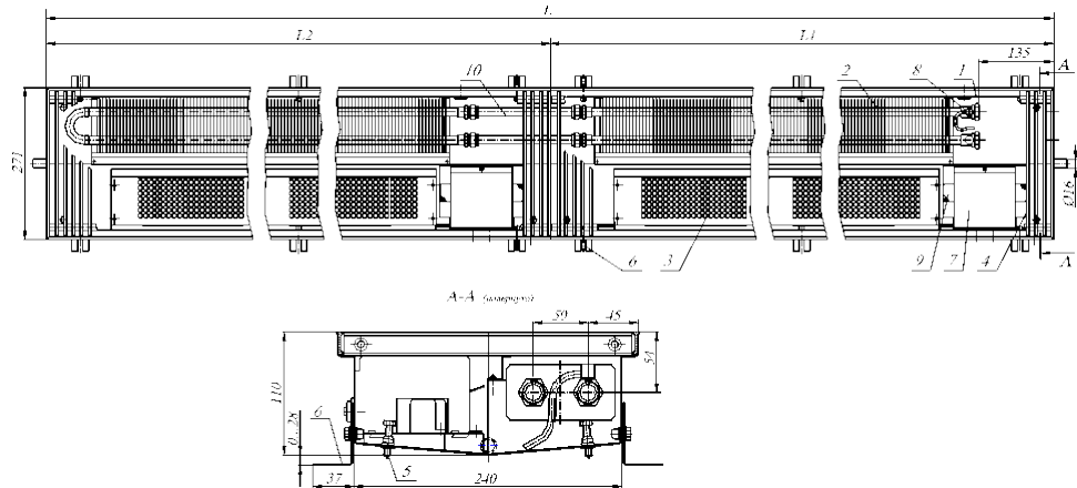
Рис.1 Конвектор КВОК12 27.11.310...600-ВКТ-П
