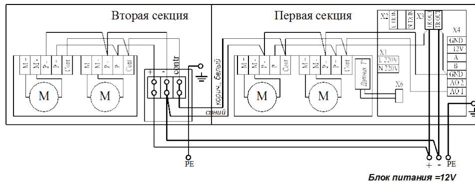
Рис. 9 Схема подсоединения электропитания конвейера «Golfstream 12VK» с контроллером Z401.
