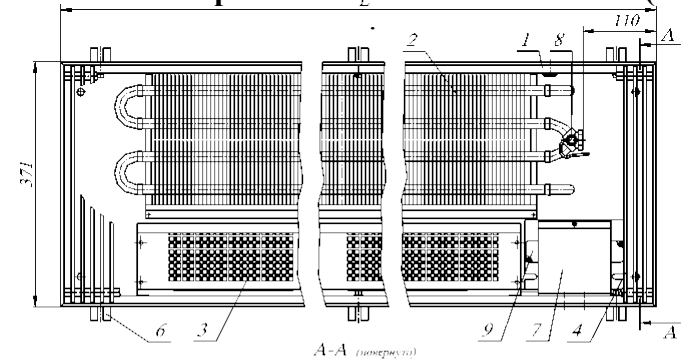
Рис.2 Конвектор КВКП12 27.14.060...300-ВК(ВКТ)-П
