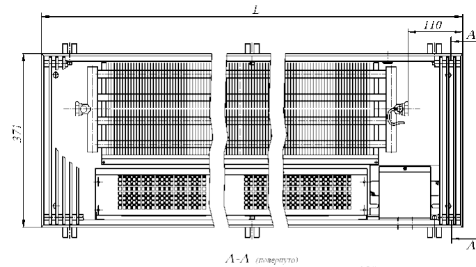
Рис.3 Конвектор КВКД12 37.14.060...300-ВК(ВКТ)-П
