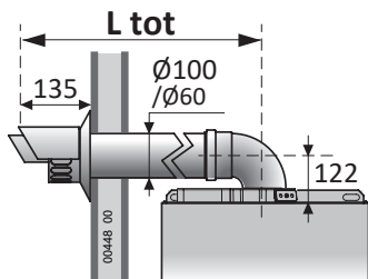
Пример горизонтальной системы «коаксиальной» (C 13 )
