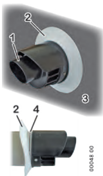
Пример горизонтальной системы «коаксиальной» (C 13 )
