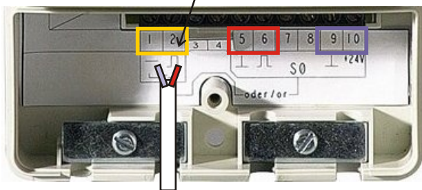
Клеммная коробка преобразователя
