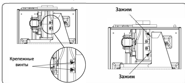
Рис. 18 – Снятие теплообменника
