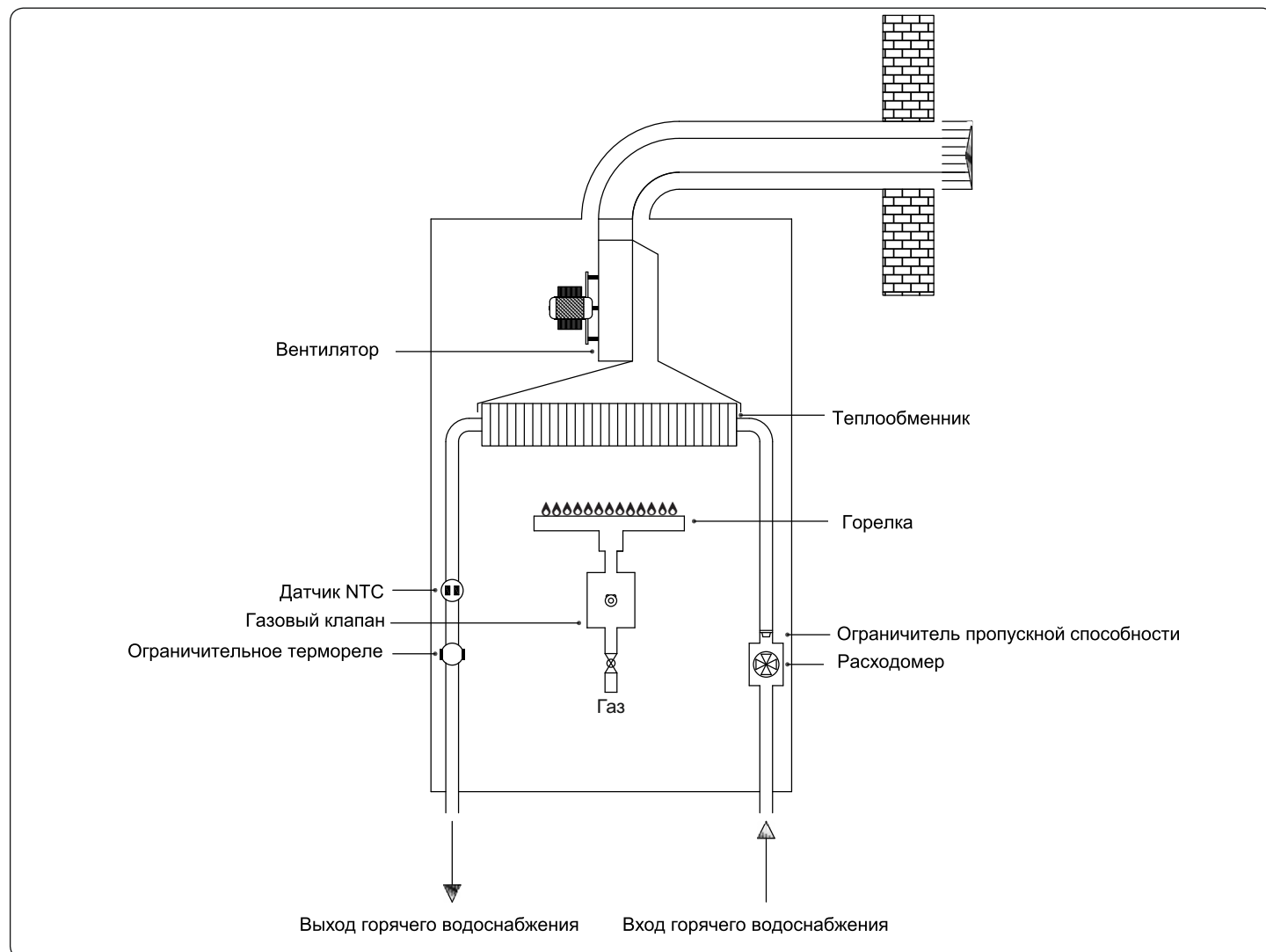
Рис. 3 – Гидравлическая сеть
