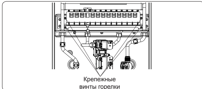
Рис. 19 – Снятие горелки
