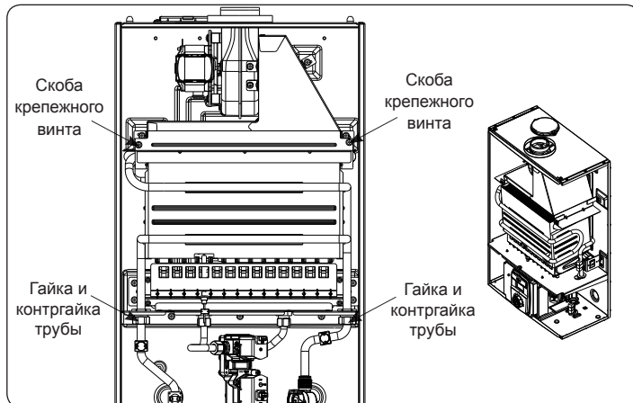
Рис. 19 – Снятие горелки
