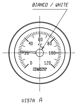
VISTA A
