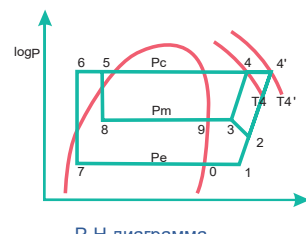
P-h диаграмма
