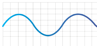
Синусоидальное управление постоянным током на 180°
