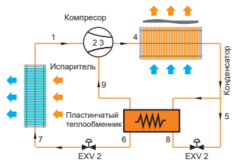
Схема фреонового контура
