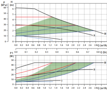
Рис.11: Характеристики насоса Alpha2L xx40
