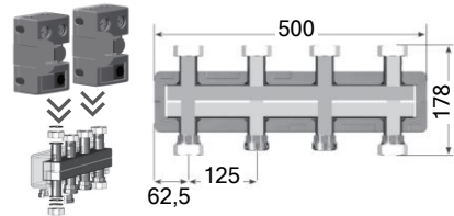
Рис 5: Распределительный коллектор
