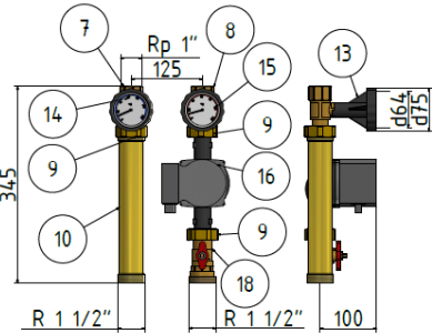
Рис.2: Прямая насосная группа DN25 ECO-2
