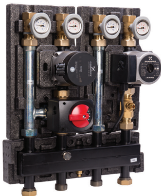
Общий вид распределительной системы ECO 2 MINI DN20 (3/4")
