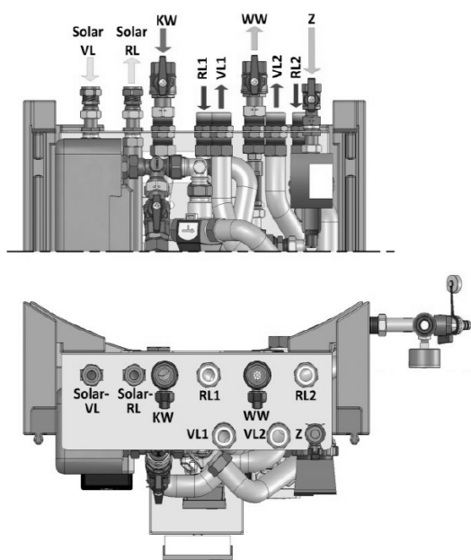
Рис. 3-11 Гидравлические подключения I
