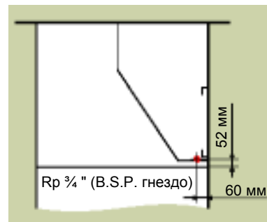
Рис.2 Местоположение и размеры отверстия
