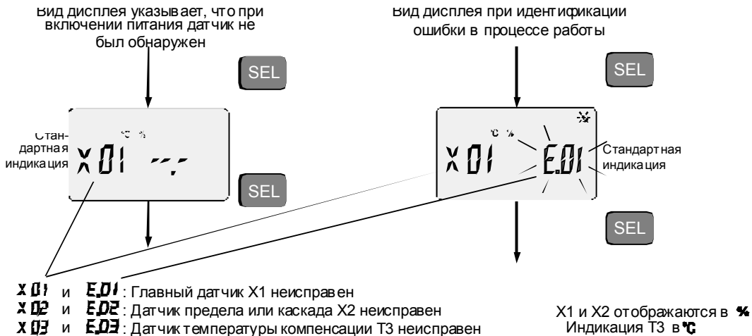
Рис. 11 Обработка ошибок
