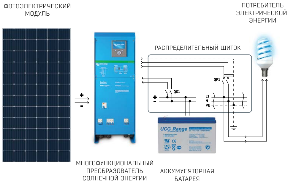
Рисунок 1.1 Блок-схема по подключению оборудования системы
