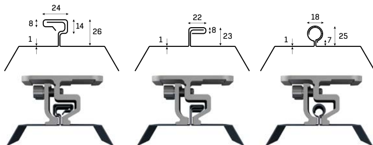
Рисунок 3.2.5 Способ крепления к фальцевой кровле
