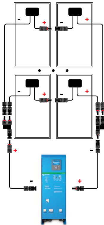
Рисунок 3.3.1.1 Схема подключения постоянного тока для комплекта A7 (6 цепочек по 2 ФЭМ)
